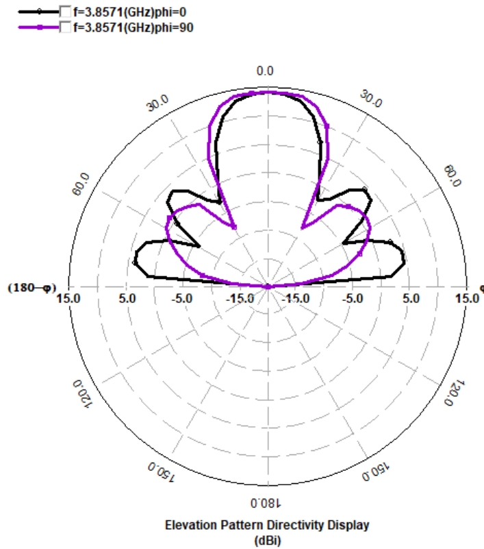
Ilustración 22: Diagrama de radiación de la estructura con un parche en IE3D
