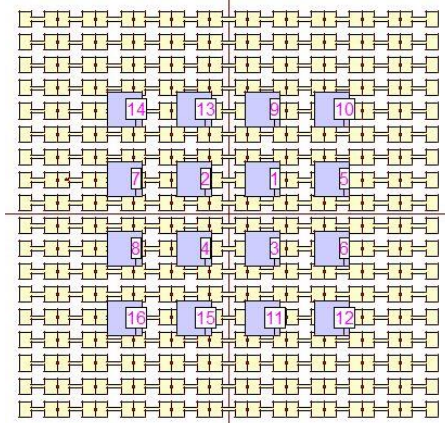
Estructura con dieciséis parches
