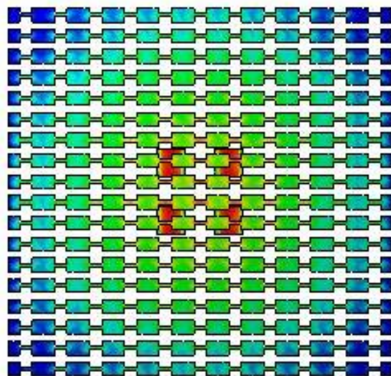
Ilustración 30: Corriente a 3,85 GHz de la estructura con cuatro parches en IE3D
