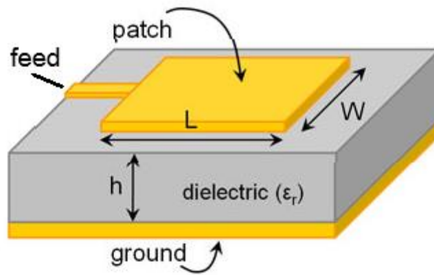
Ilustración 2: Estructura de una antena microstrip
