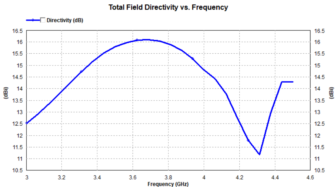
Ilustración 41: Directividad de la estructura con dieciséis parches en IE3D
