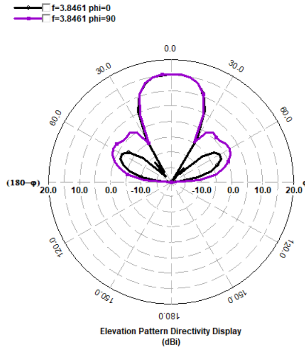
Ilustración 32: Diagrama de radiación de la estructura con cuatro parches en IE3D
