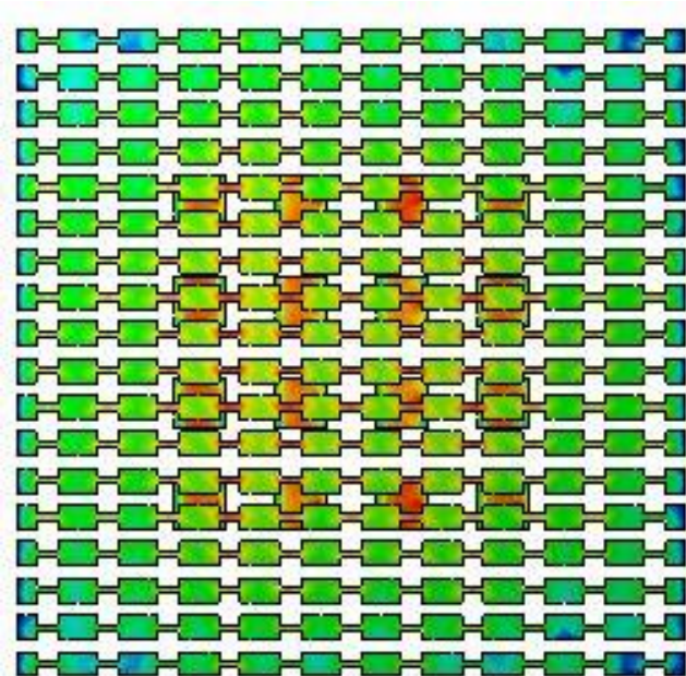
Ilustración 40: Corriente a 3,85 GHz de la estructura con dieciséis parches en IE3D
