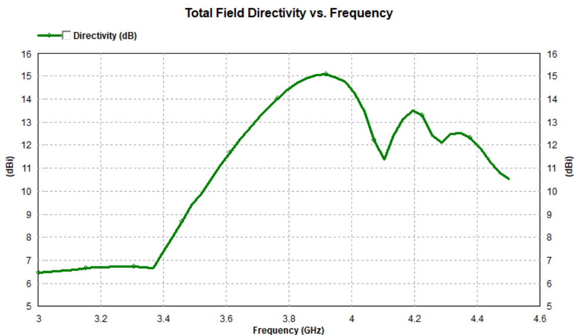
Ilustración 26: Directividad de la estructura con dos parches en IE3D
