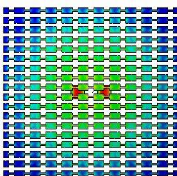
Ilustración 25: Corriente a 3,85 GHz de la estructura con dos parches en IE3D
