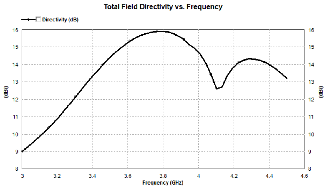
Ilustración 36: Directividad de la estructura con ocho parches en IE3D
