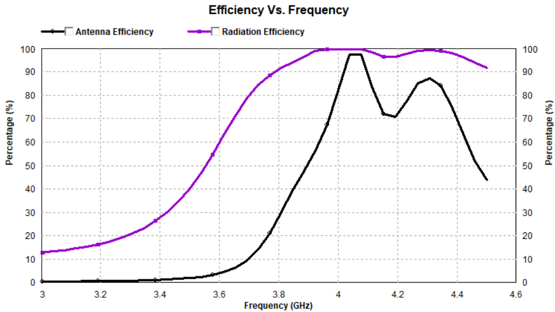
Ilustración 33: Eficiencia de antena y de radiación de estructura con cuatro parches en IE3D
