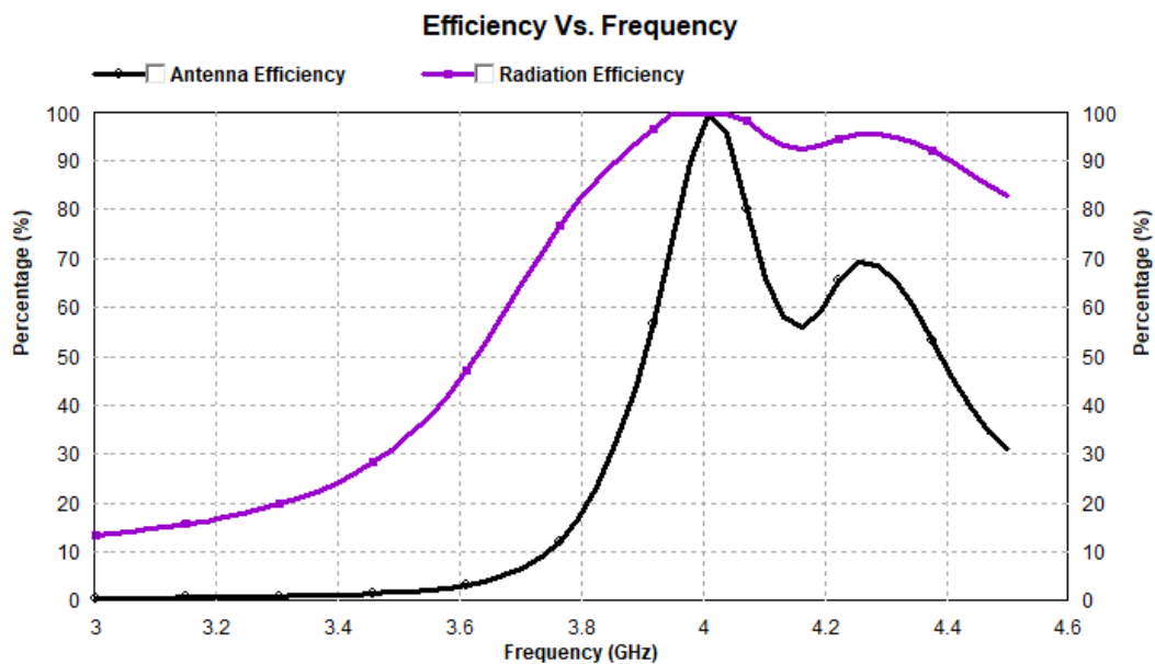
Ilustración 28: Eficiencia de antena y de radiación de estructura con dos parches en IE3D
