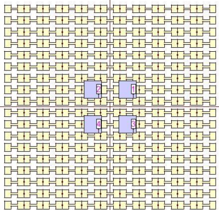
Estructura con cuatro parches
