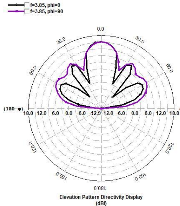
Ilustración 47: Diagrama de radiación de la estructura con treinta y dos parches en IE3D
