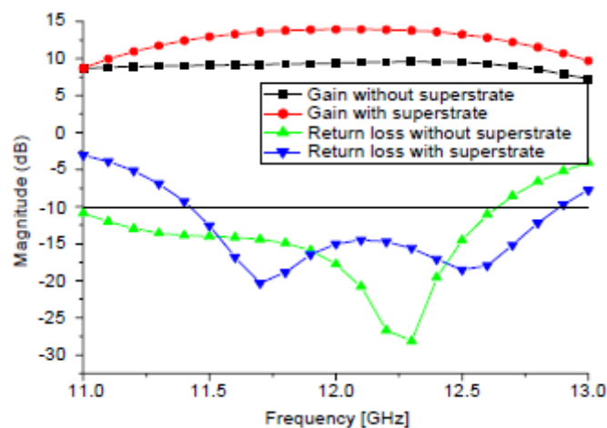
Ilustración 15: Resultados simulados con y sin el superestrato
