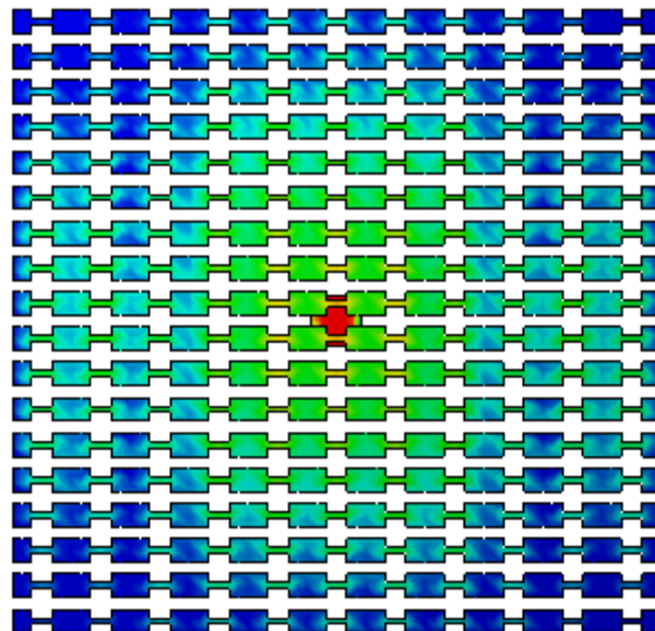
Ilustración 20: Corriente a 3,85 GHz de la estructura con un parche en IE3D
