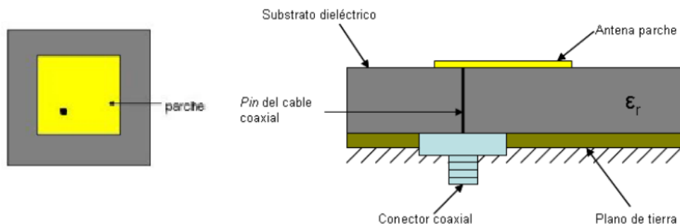
Ilustración 3: Antena microstrip alimentada por sonda coaxial
