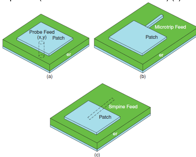
Ilustración 7: Técnicas de alimentación de antenas microstrip
