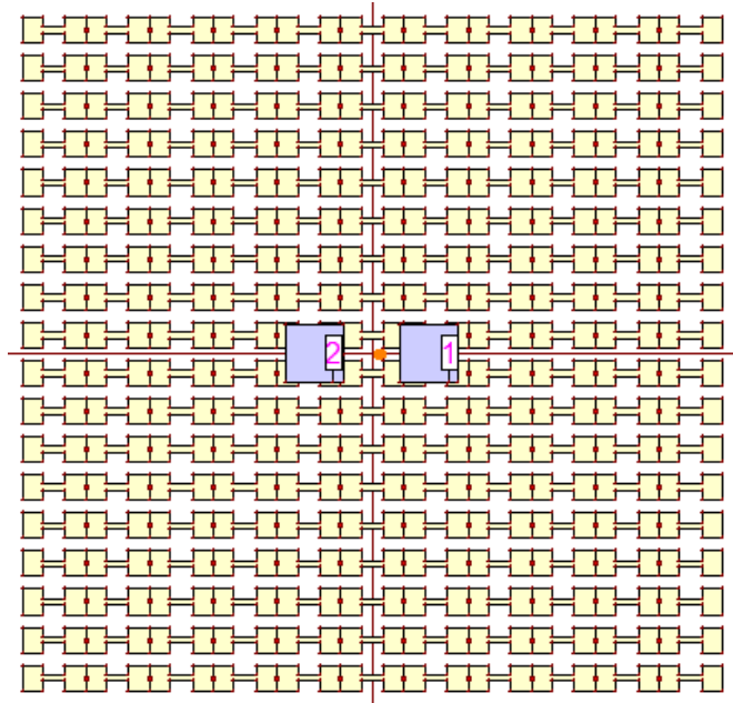
Ilustración 24: Estructura con dos parches en IE3D
