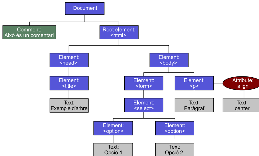
Figura 8. Exemple d'arbre HTML
