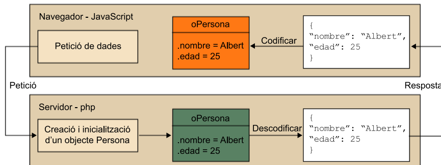
Figura 15. Codificació i descodificació de dades JSON
