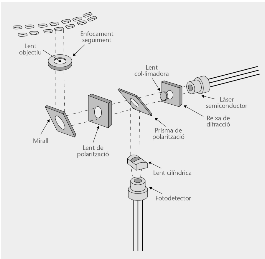
Figura 9. Distribució de lents, prismes i sensors que intervenen en el procés de lectura d'un disc òptic
