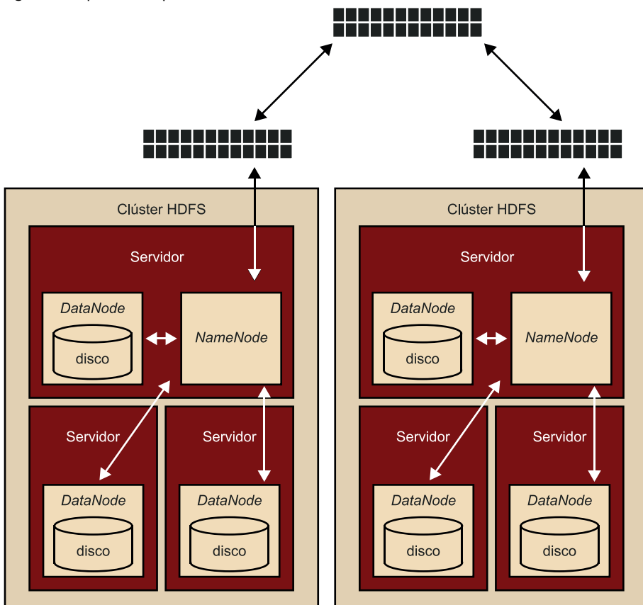
Figura 8. Arquitectura típica de un clúster HDFS
