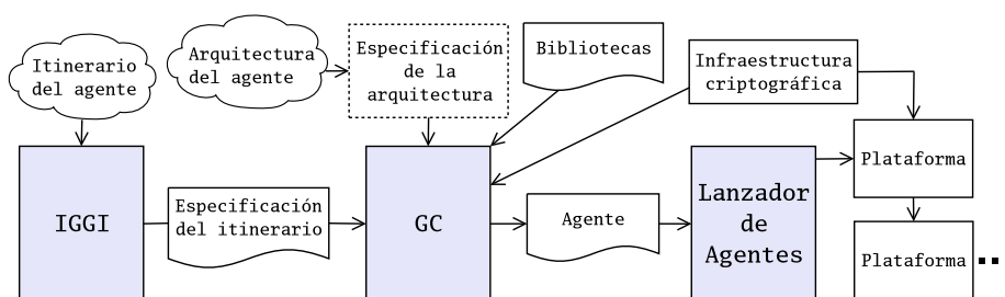
Figura 1. Componentes del esquema de desarrollo
