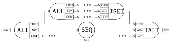
Figura3. Bloques de código de un itinerario genérico.
