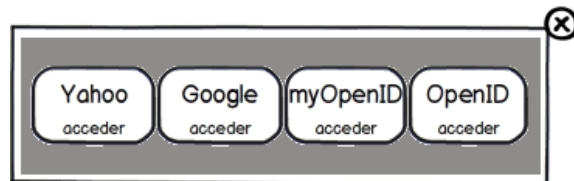
Ilustración 2: Identificación OpenID
