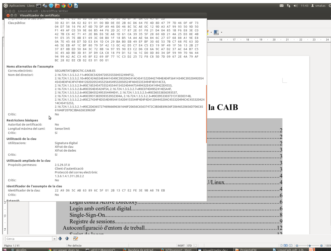
Figura 3: error gcr-viewer
