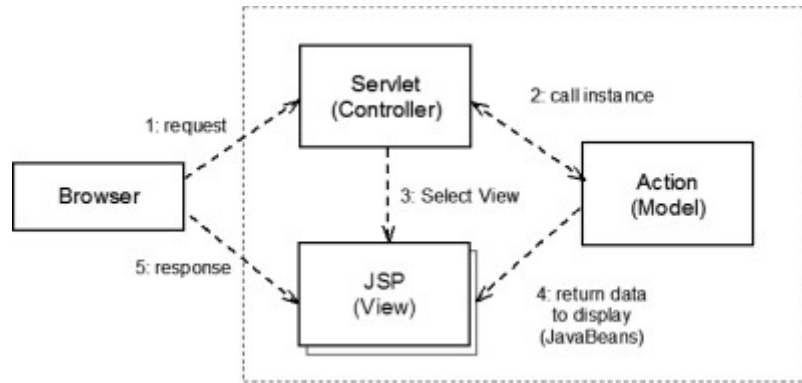
Gràfic 15. Interacció tecnologia JSP
