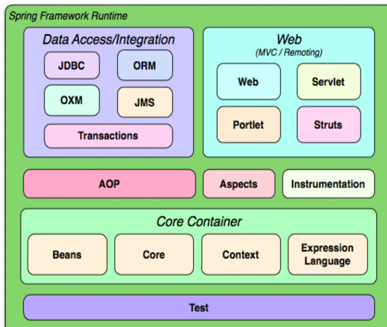
Gràfic 14. Components framework Spring
