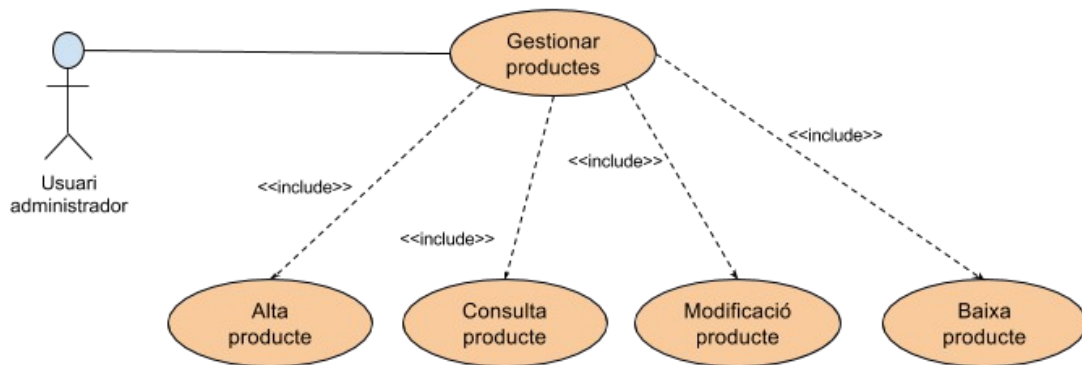
Gràfic 6. Diagrama de cas d'ús gestionar productes
