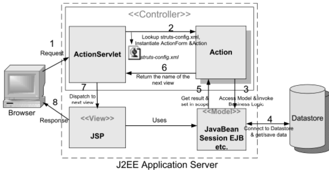
Gràfic 16. Arquitectura aplicació struts
