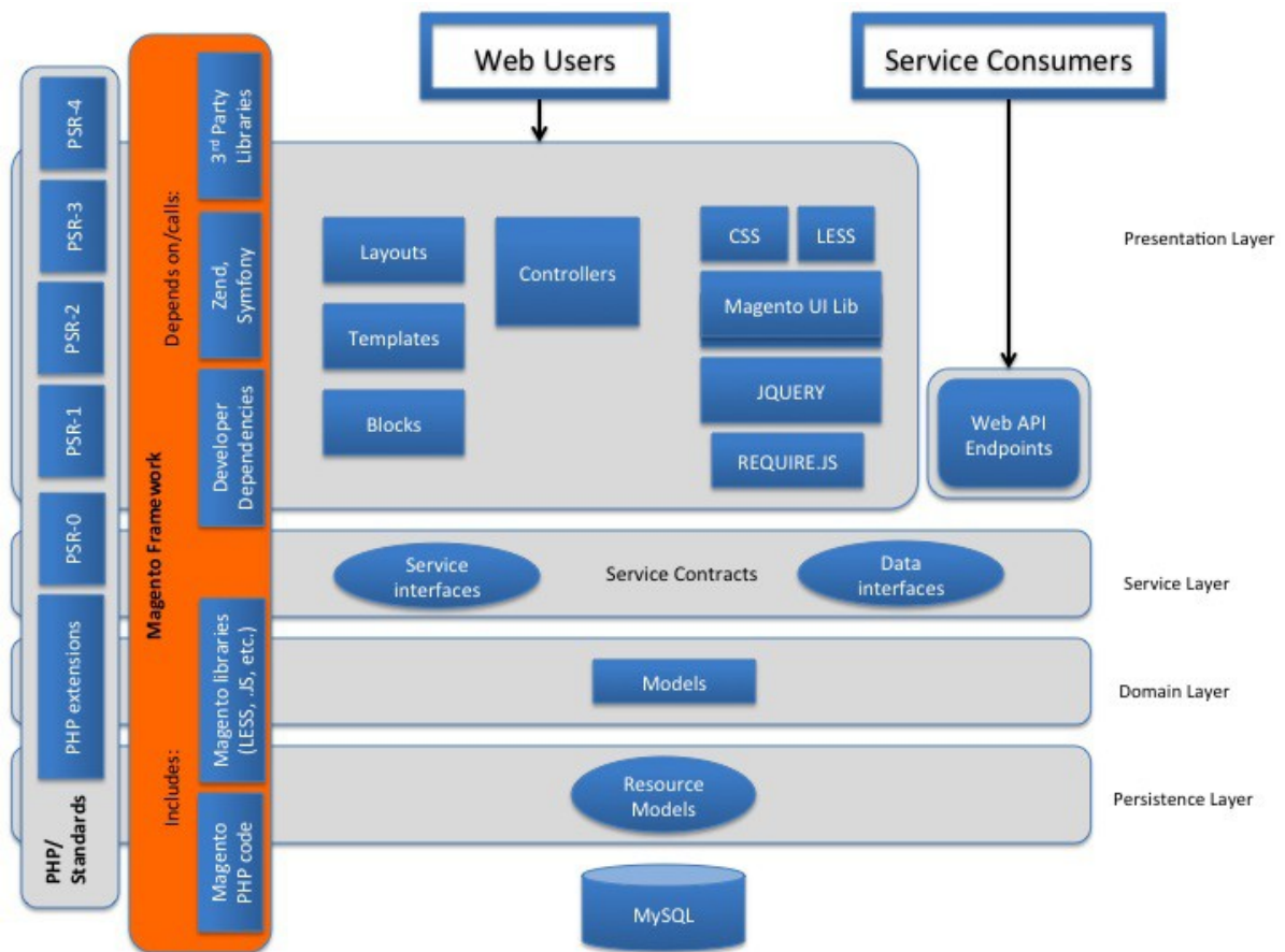
Gràfic 17. Arquitectura magento
