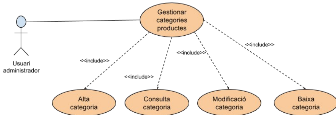
Gràfic 7. Diagrama de cas d'us gestionar categories productes
