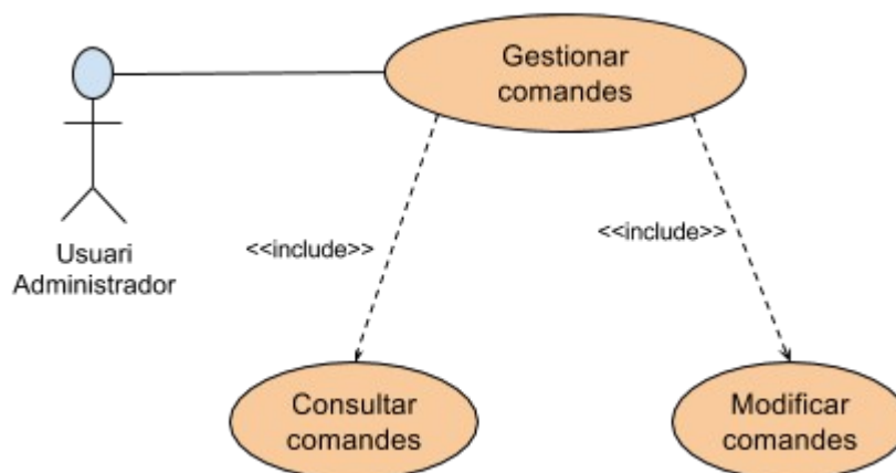
Gràfic 9. Diagrama de cas d'us gestionar comandes
