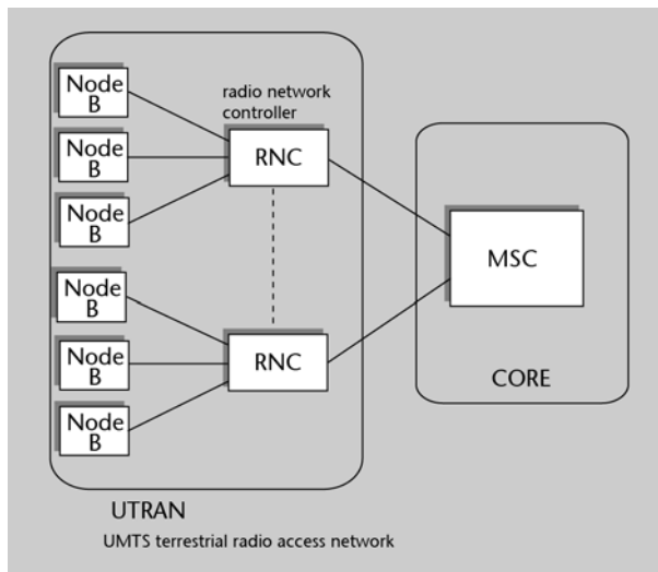
Arquitectura UMTS bàsica
