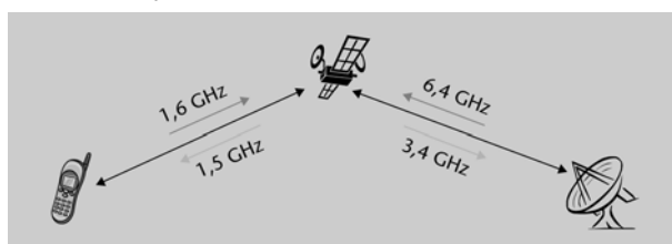
Sistema Thuraya
