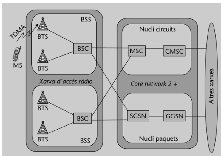
Arquitectura GSM/GPRS
