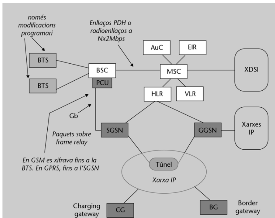
Arquitectura GPRS
