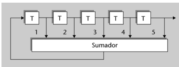
Connexions genèriques
