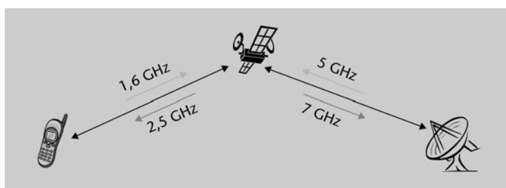
Globalstar
