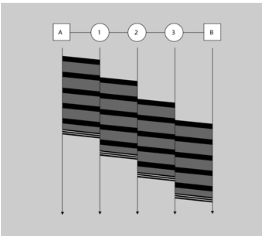
Figura 8. Diagrama temporal d'una connexió en mode datagrama
