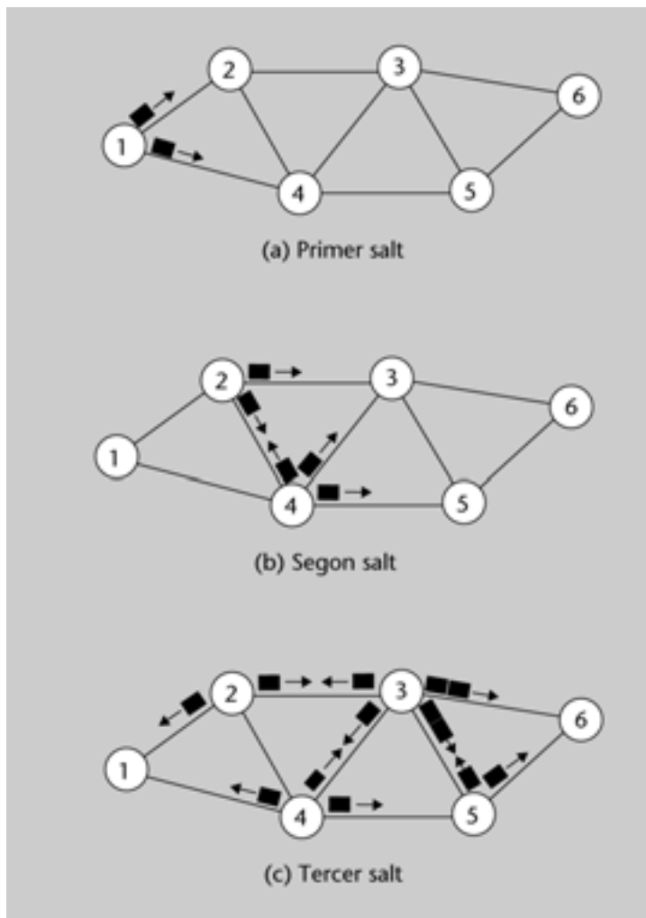
Figura 12. Encaminament per flooding . Inundació de la xarxa amb rèpliques
