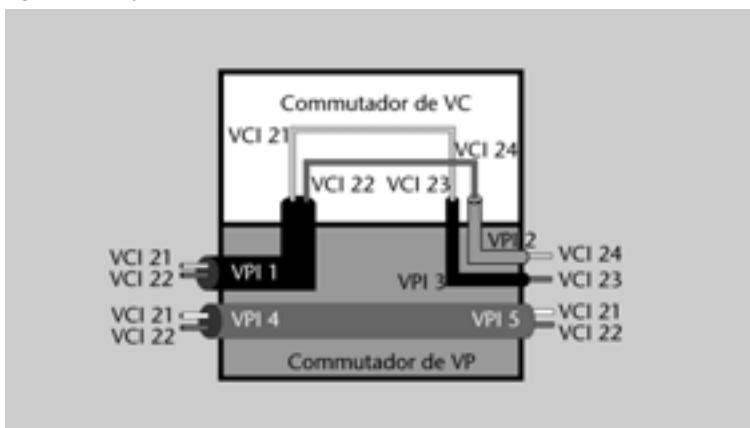
Figura 36. Esquema de commutació dels canals virtuals
