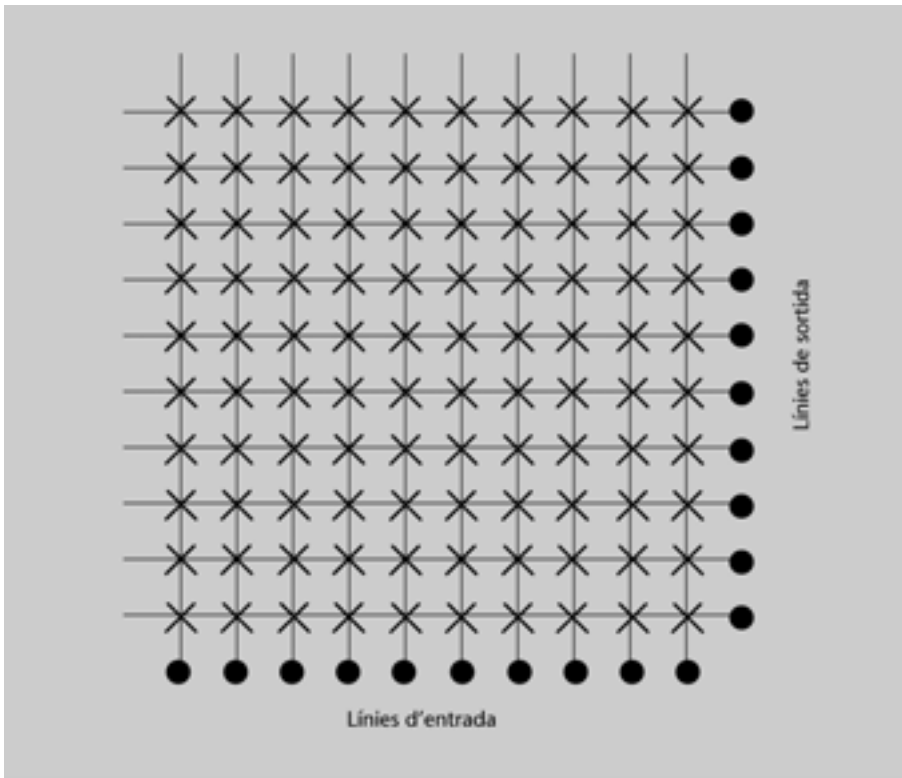
Figura 17. Xarxa de commutació formada per una matriu de commutadors
