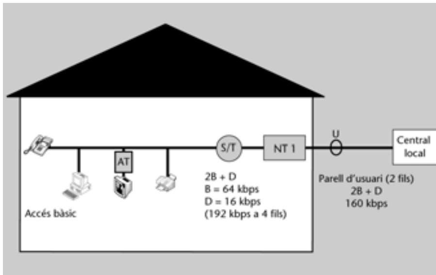
Figura 23. Accés bàsic (BRI) a la XDSI
