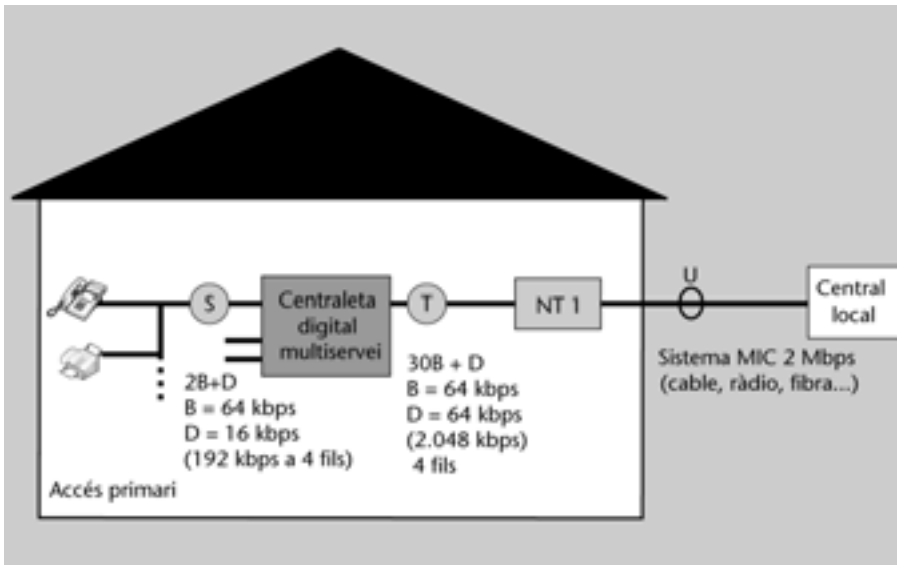
Figura 24. Accés primari (PRI) a la XDSI
