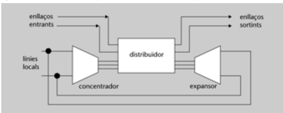
Figura 18. Commutador multietapa: concentració, distribució i expansió
