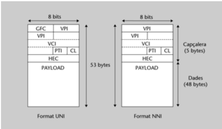
Figura 33. Format dels dos tipus de cel·les ATM
