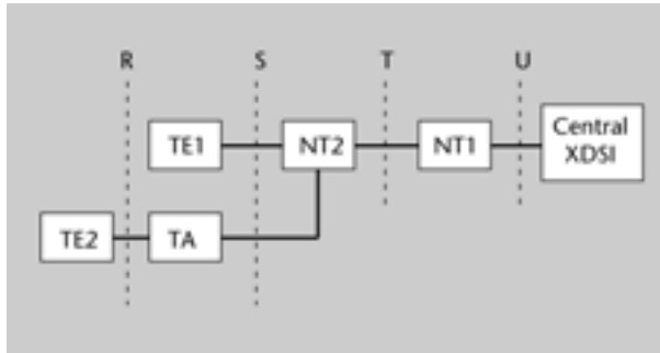
Figura 22. Configuració de referència de l'accés d'usuari a la XDSI
