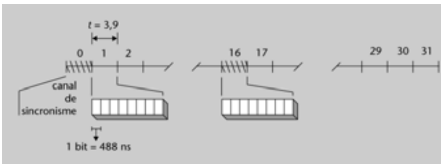
Figura 16. Representació de la trama E1
