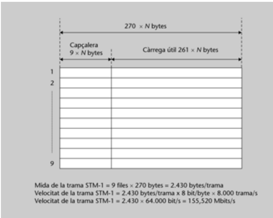
Figura 31. Estructura de la trama STM-1
