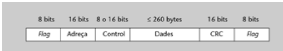
Figura 25. Estructura de la trama LAPD
