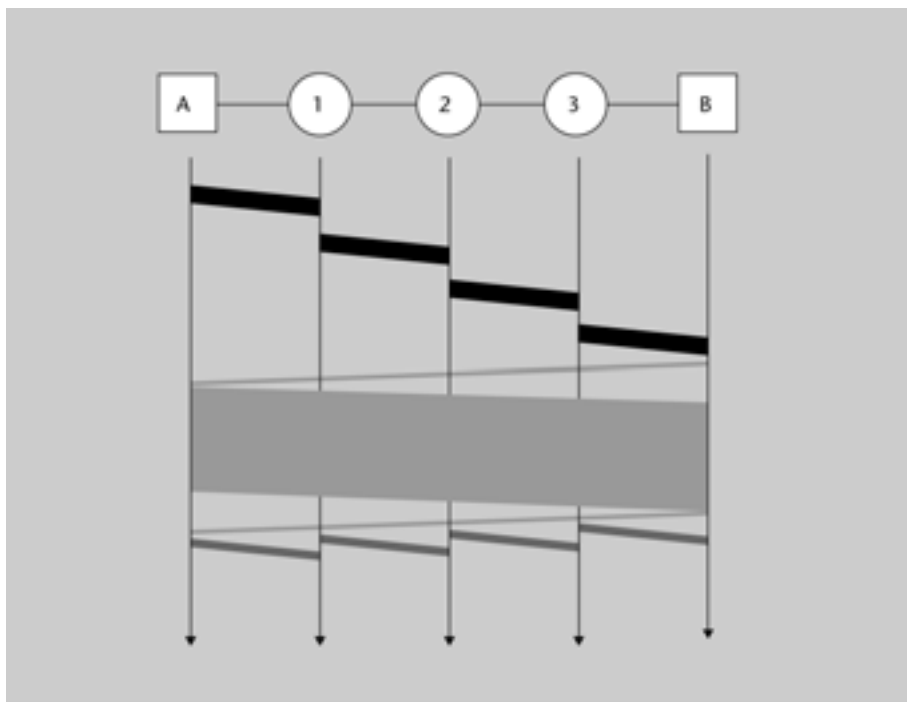
Figura 4. Diagrama temporal d'una connexió amb commutació de circuits
