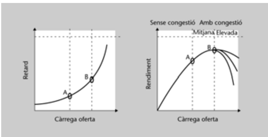
Figura 28. Efectes de la congestió sobre el retard i el rendiment
