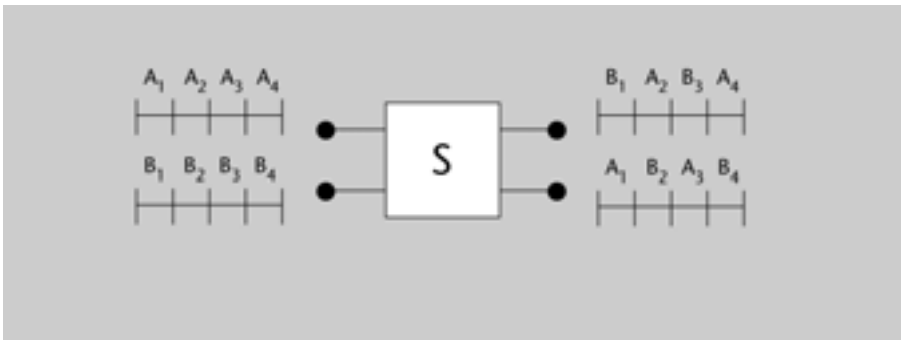
Figura 19. Commutador espacial de dues trames de quatre unitats de temps
