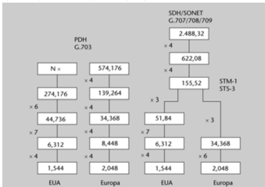
Figura 32. Esquema de les jerarquies de multiplexatge
