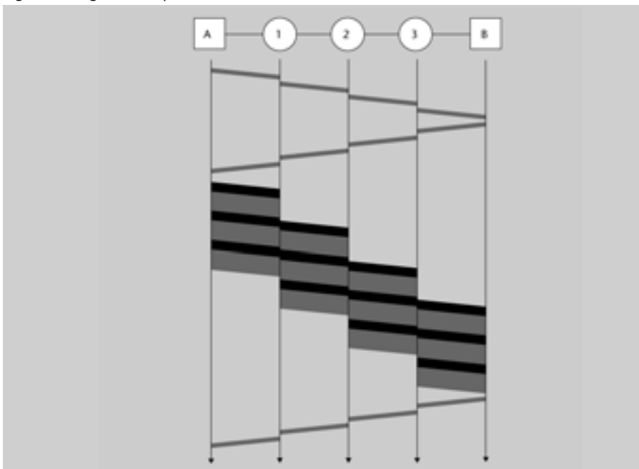
Figura 9. Diagrama temporal d'una connexió en mode circuit virtual
