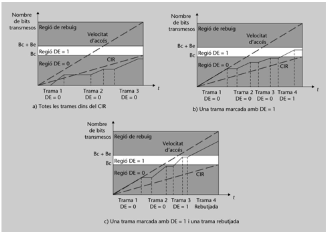
Figura 29. Exemples de gestió del trànsit
