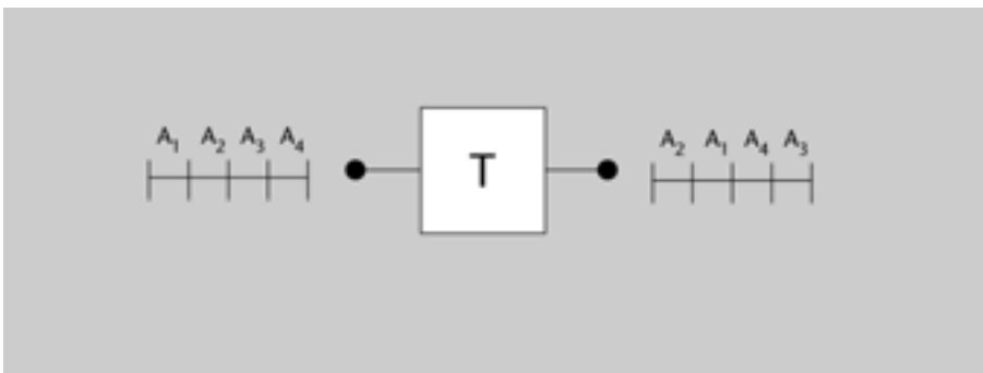
Figura 20. Commutador temporal d'una trama de quatre unitats de temps
