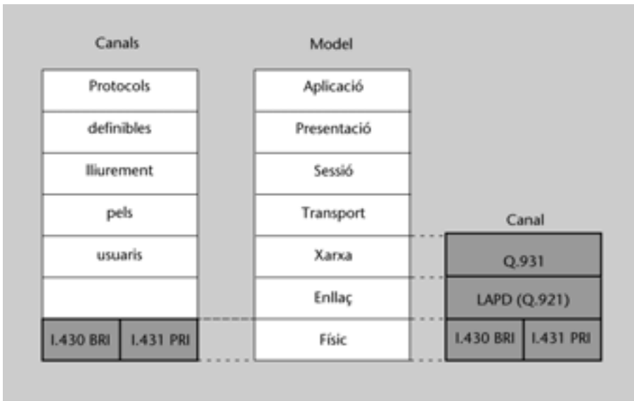
Figura 21. Equivalència entre els nivells del model OSI i l'arquitectura XDSI
