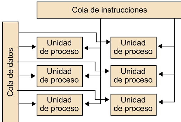
Figura 7. Múltiples instrucciones, múltiples datos
