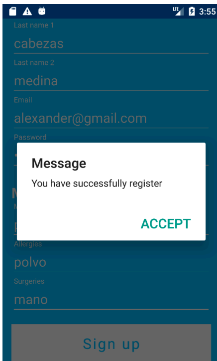
Ilustración 3. Registro exitoso
