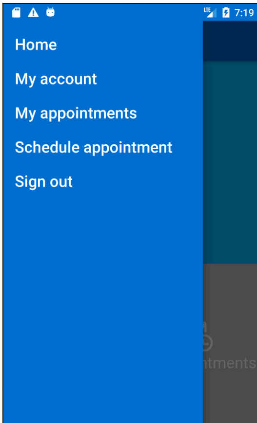
Ilustración 7. Menú lateral
