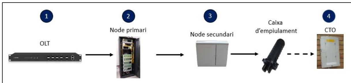
Il·lustració 6-Estructura de la xarxa
