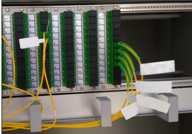
Il·lustració 10-Repardidor amb slots, raspall i fuetons
