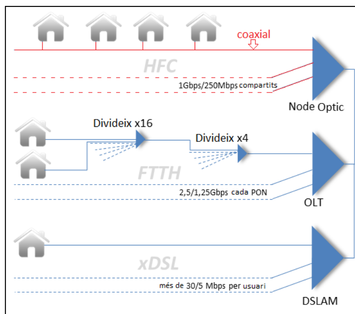
Il·lustració 2- Tipus de tecnologies de xarxes fins a client
