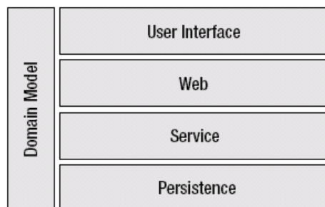
Figura 32. Capes estructurals d'Spring MVC.
