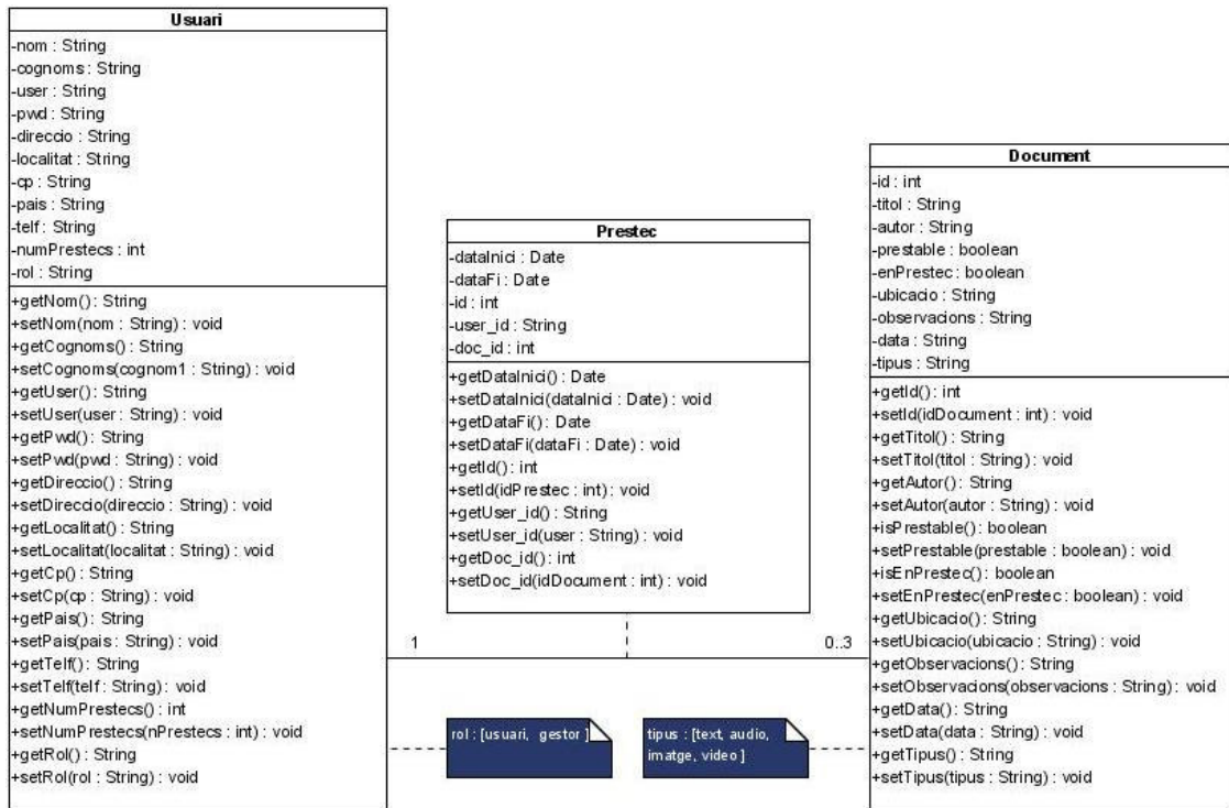
Figura 51. Diagrama de classes: escenari general modificat.
