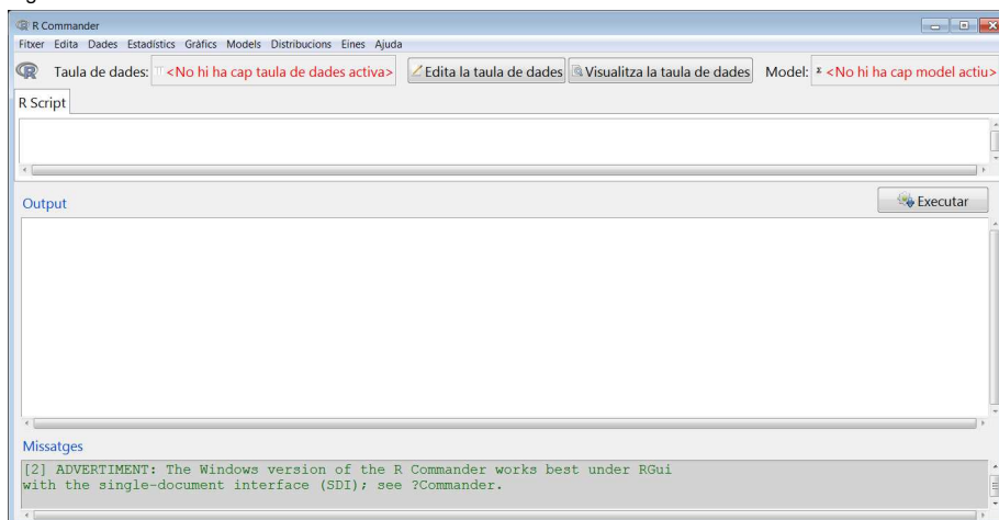
Figura 1: Interfície d'R-Commander
