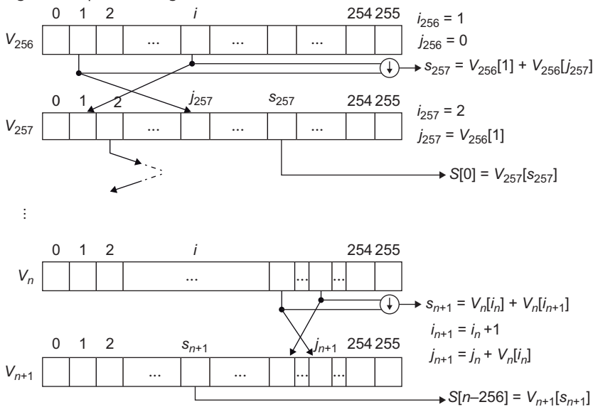
Figura 6. Esquema del algoritmo PRGA del cifrado RC4
