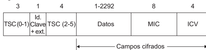
Figura 15. Datos de una trama TKIP
