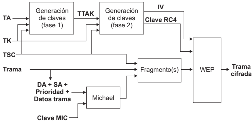
Figura 14. Generación de tramas cifradas TKIP
