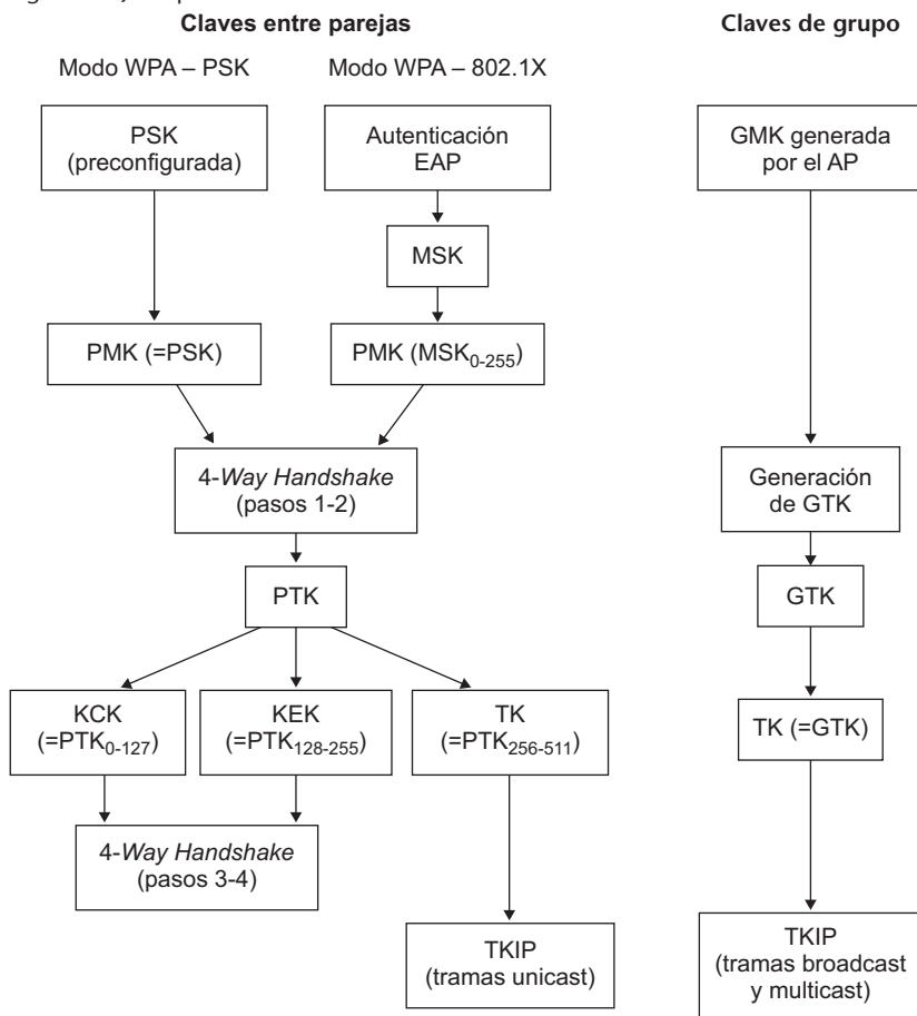
Figura 13. Jerarquía de claves WPA
