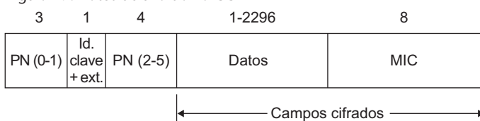
Figura 17. Datos de una trama CCMP
