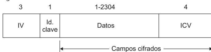
Figura 4. Datos de una trama WEP
