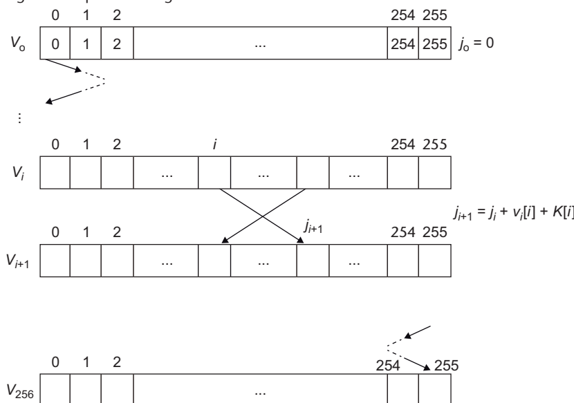
Figura 5. Esquema del algoritmo KSA del cifrado RC4
