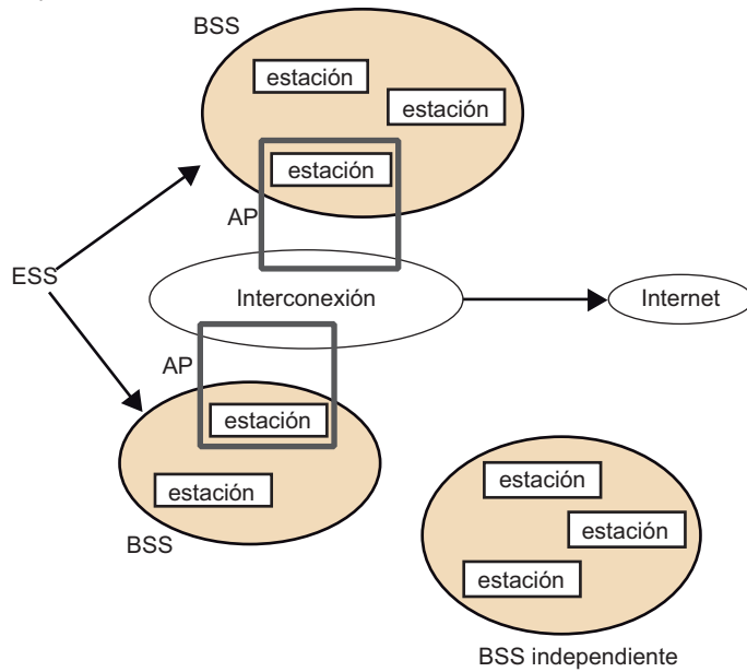
Figura 1. Componentes de las redes Wi-Fi
