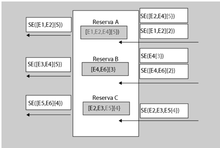
Figura 9. Ejemplo de reserva en un encaminador con estilo de filtro explícito compartido, SE
