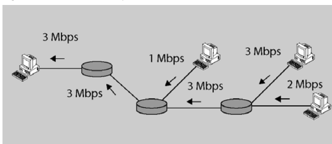
Figura 6. Fusión de los flujos en RSVP
