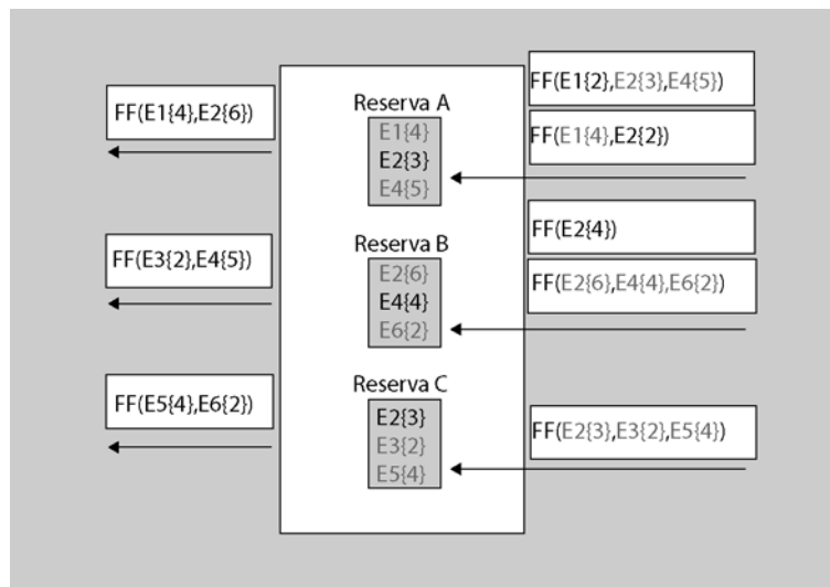
Figura 8. Ejemplo de reserva en un encaminador con estilo de filtro fijo, FF
