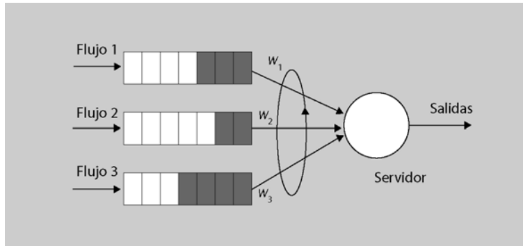
Figura 3. Modelo de disciplina de planificación de enlace equitativo ponderado
