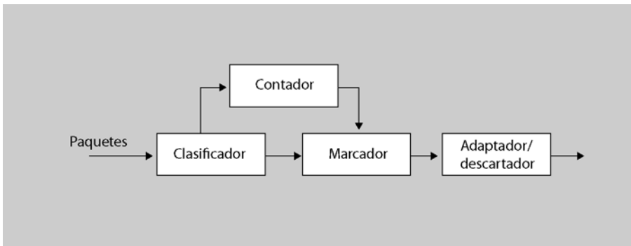
Figura 11. Elementos de un acondicionador de tráfico
