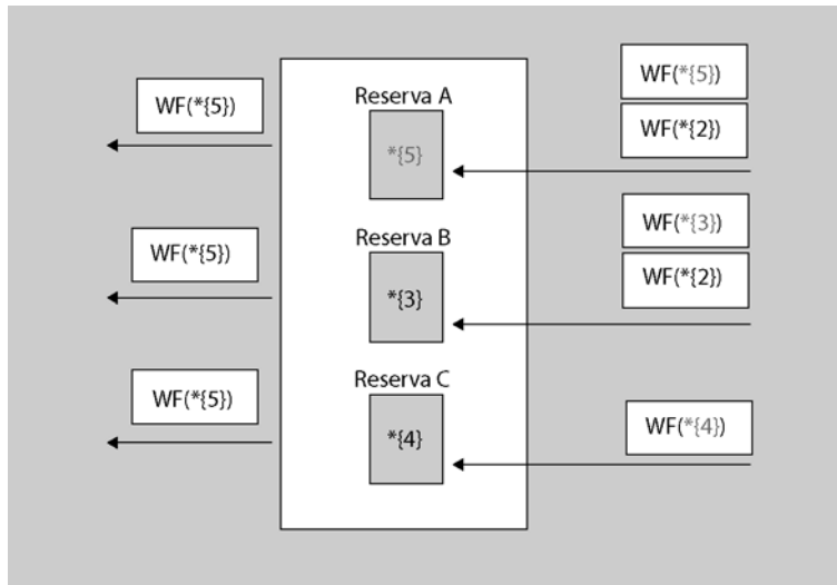
Figura 7. Ejemplo de reserva en un encaminador con estilo de filtro comodín, WF
