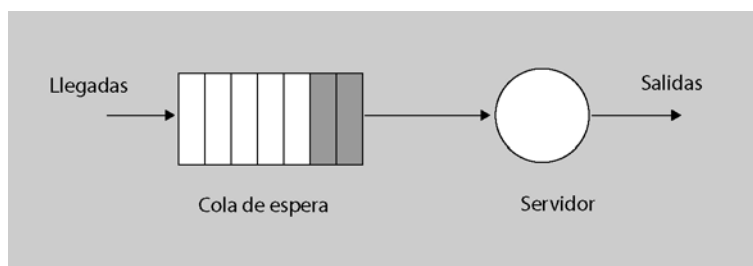
Figura 1. Modelo de disciplina de planificación de enlace FIFO
