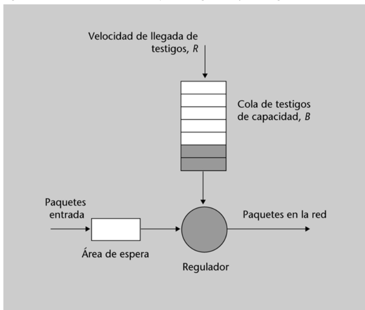
Figura 4. Modelo de control de flujo con regulador por testigos
