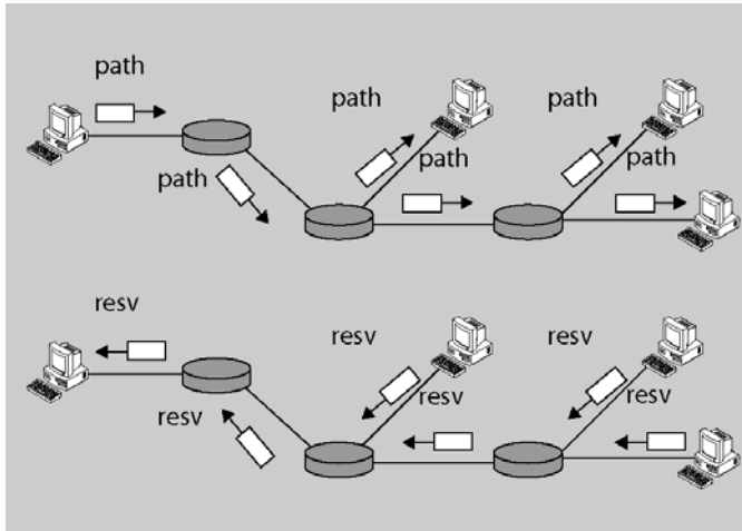
Figura 5. Envío de mensajes para establecer un camino
