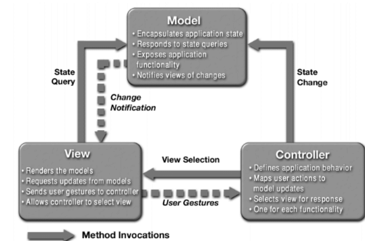
ILUSTRACIÓN 35. DIAGRAMA MVC
