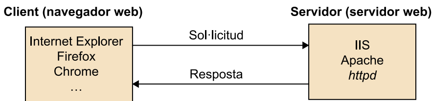
Figura 48. Arquitectura client-servidor
