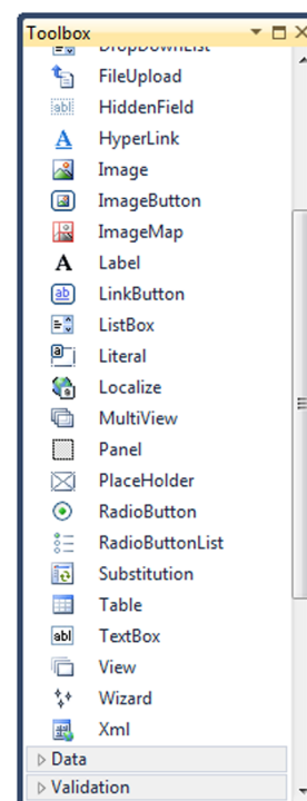
Figura 17. Quadre d'eines
