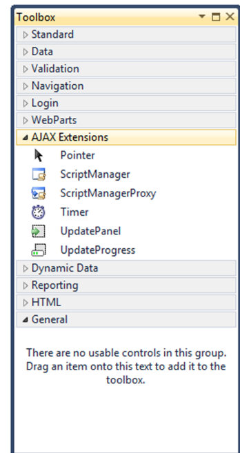
Figura 99. Caixa d'eines
