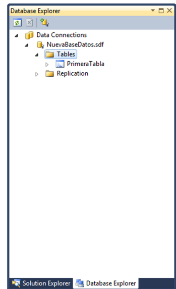
Figura 31. Nova taula
