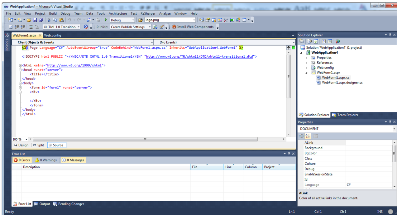
Figura 8. Visual Studio 2010
