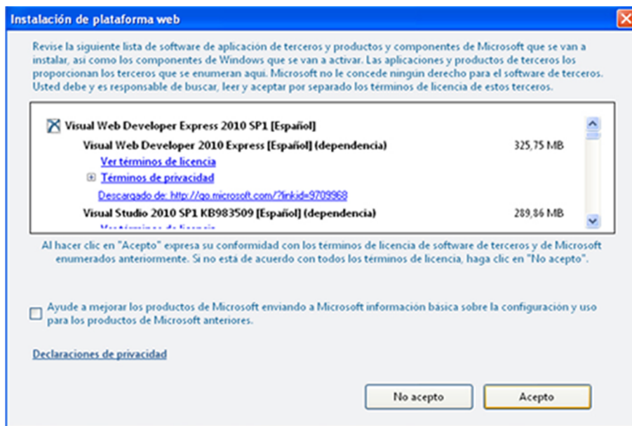
Figura 12. Condicions d'ús
