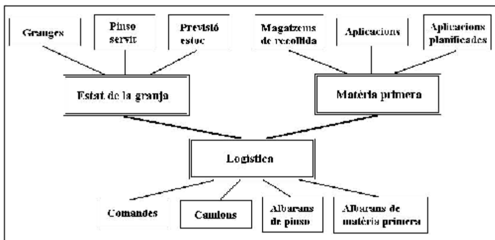
Figura 22 . Estructura de la base de dades de logística
