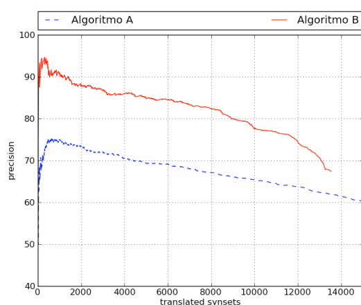
Figura 3: Comparación de los algoritmos A y B para el catalán.
