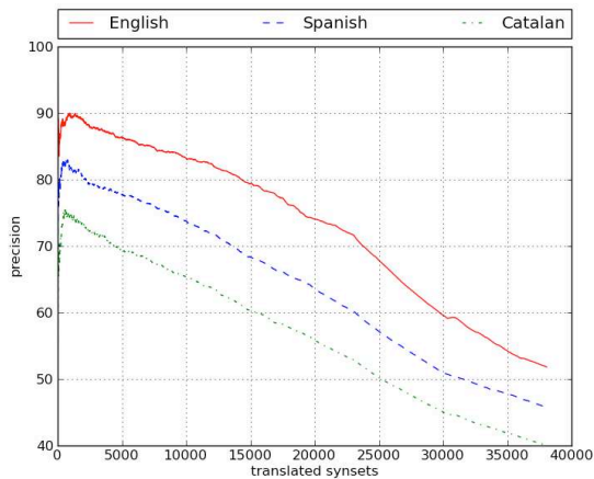
Figura 1: Comparación de los resultados del algoritmo A para el inglés, castellano (Google) y catalán (Google).
