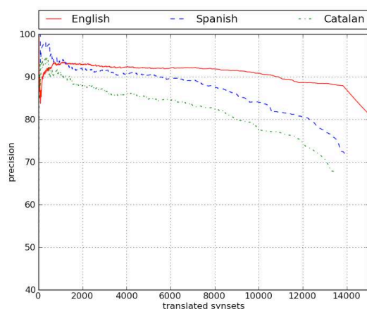
Figura 2: Resultados correspondientes al algoritmo B para el inglés, español y catalán.
