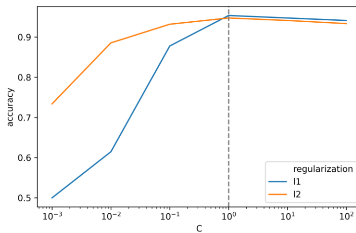
Figura 18. Evolució de l' accuracy de la logistic regression en el conjunt de validació segons el cost de regularització ( C ) i el tipus de regularització.
