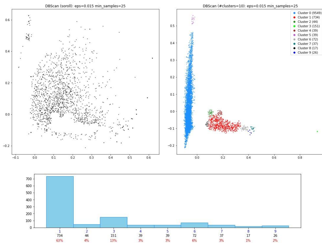
Figura N° 54: Agrupament per DBSCAN amb paràmetres eps=0.015 i min_samples=25.
