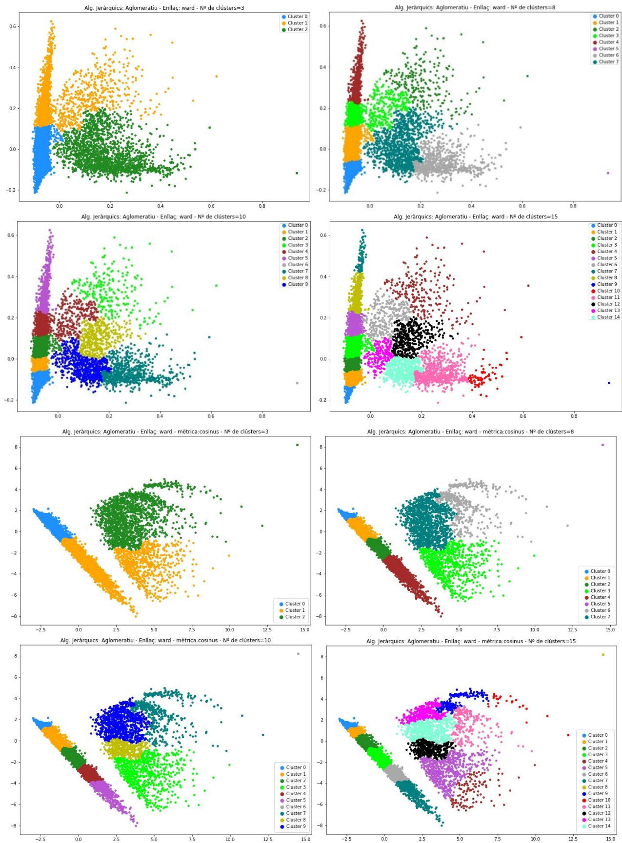
Figura Nº 71: Comparativa entre clústers amb mètrica euclidiana i similitud del cosinus (enllaç ward).
