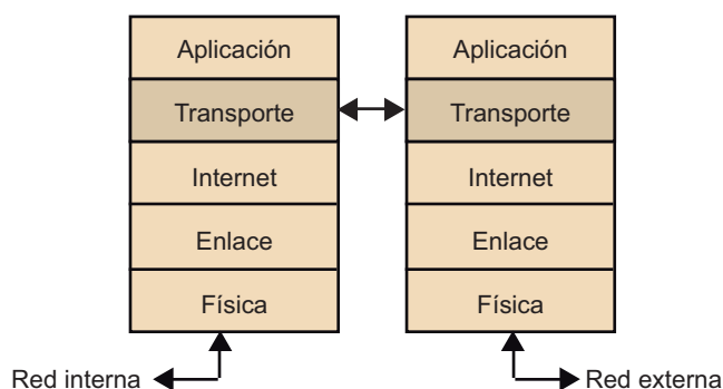
Figura 2. Pasarela a nivel de circuito
