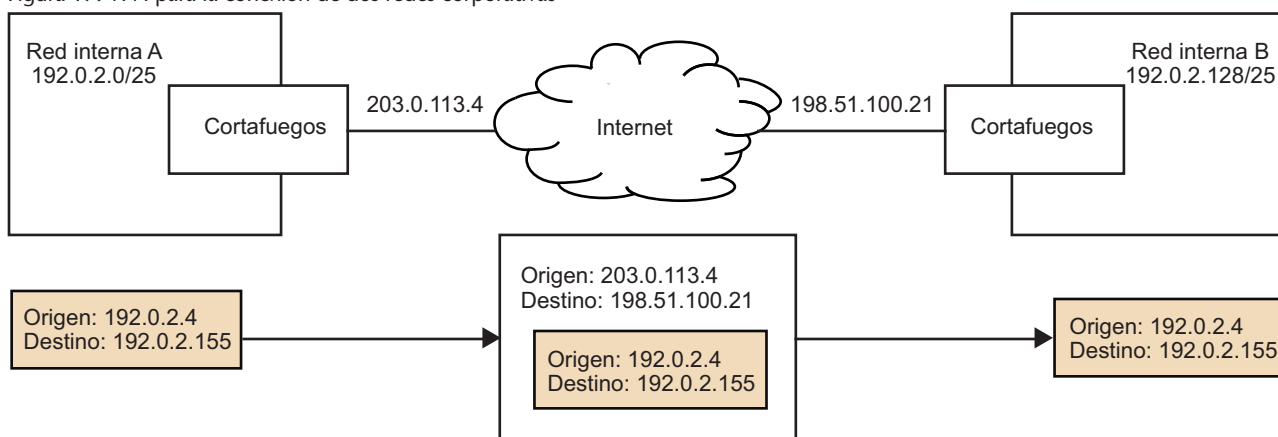
Figura 17. VPN para la conexión de dos redes corporativas
