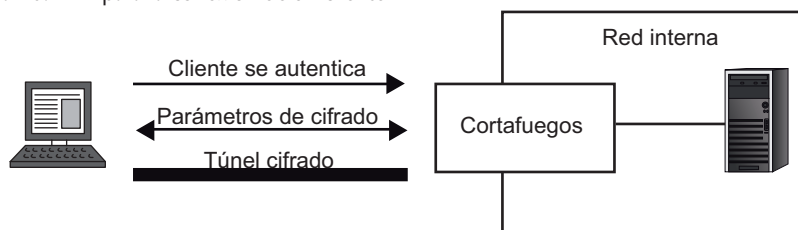
Figura 16. VPN para la conexión de un cliente
