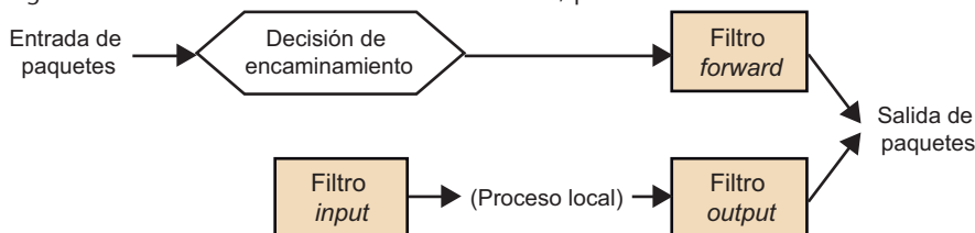
Figura 12. Cadenas de la tabla de filtrado de Netfilter/iptables
