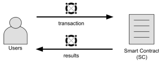
Figura 18: Requisit funcional 10.
