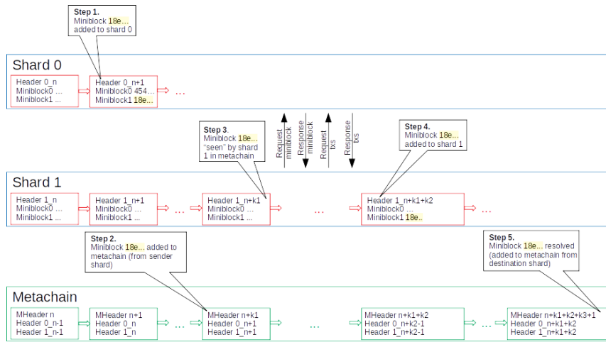
Figura 7: Exemple d’execució de transacció entre dos shards . (Font: Fig. 4 de [2]).
