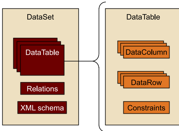
Figura 3. Estructura de un DataSet
