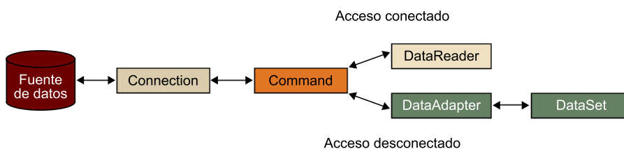
Figura 2. Modos de acceso de ADO.NET
