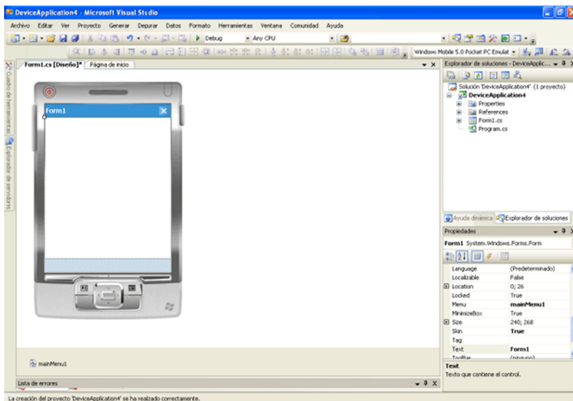
Figura 36. Diseñador de WinForms para dispositivos móviles
