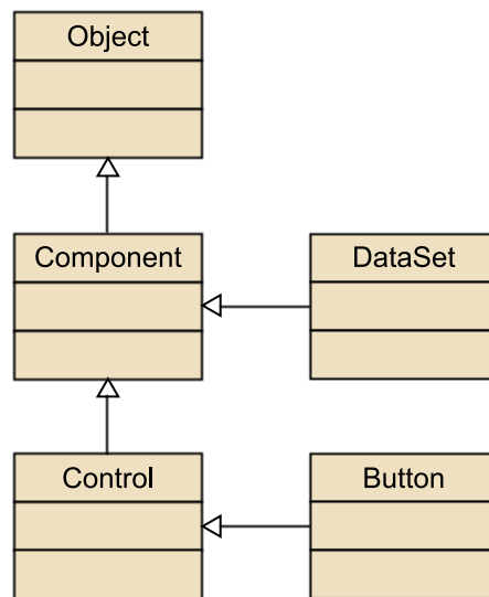
Figura 8. Jerarquía simplificada de componentes y controles
