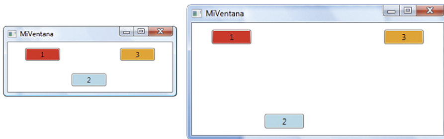
Figura 14. Ejemplo de panel Canvas
