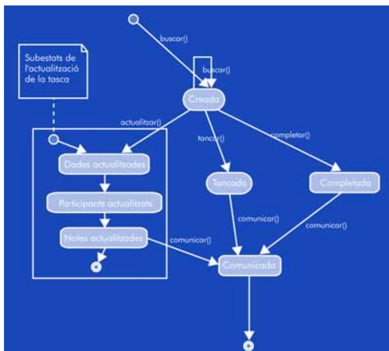
Figura 35. Diagrama d'estats amb un subestat
