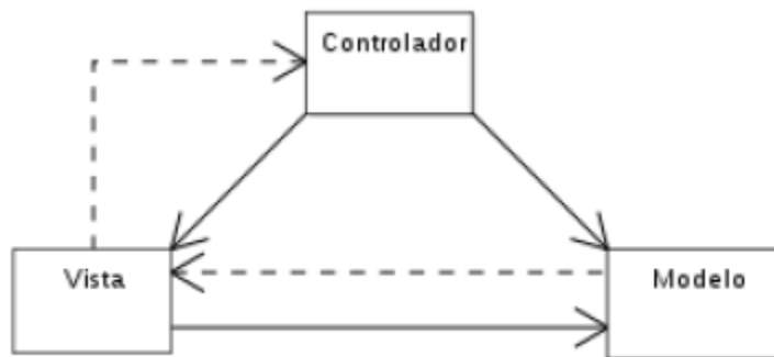
Arquitectura MVC tradicional
