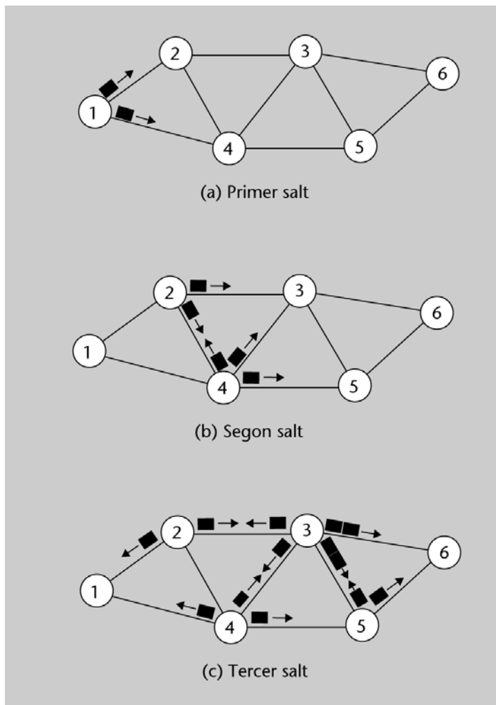
Figura 10. Encaminament per flooding . Inundació de la xarxa amb rèpliques
