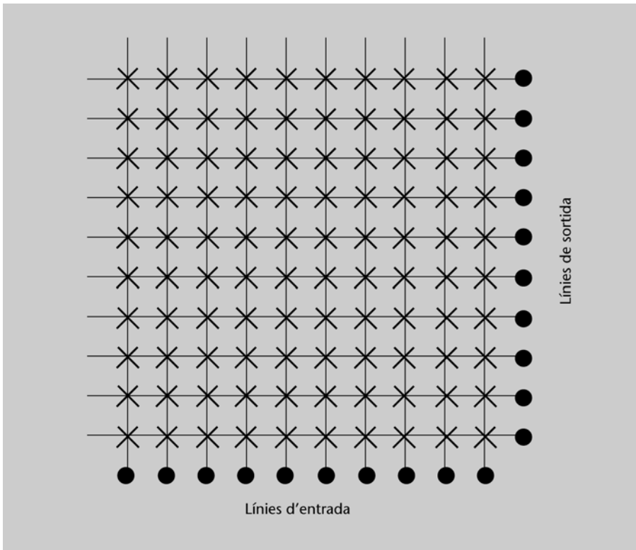
Figura 15. Xarxa de commutació formada per una matriu de commutadors
