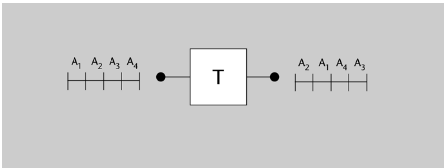
Figura 18. Commutador temporal d'una trama de quatre unitats de temps
