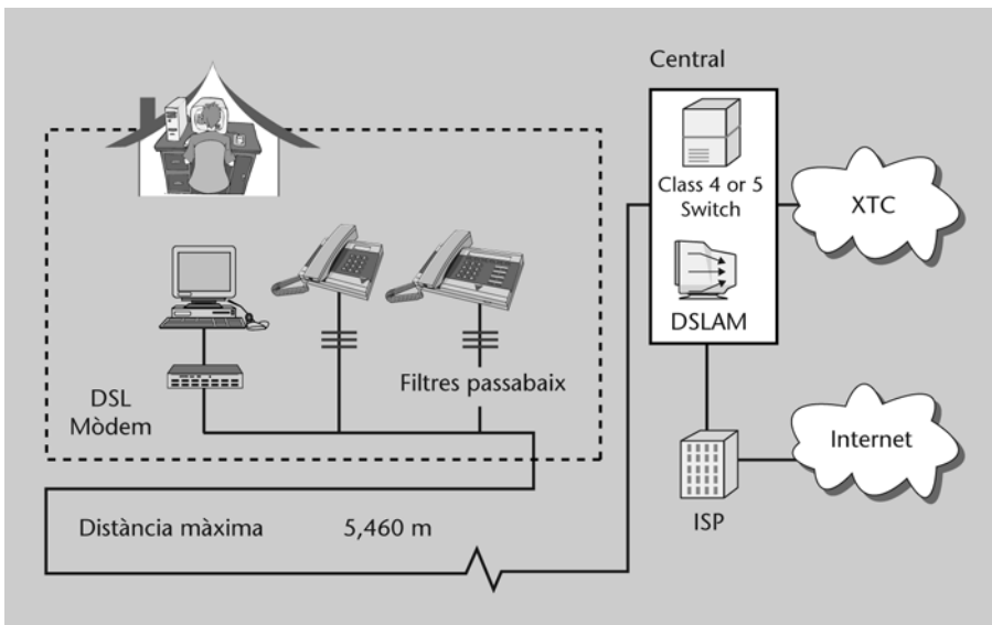
Figura 20. Elements d'una connexió ADSL
