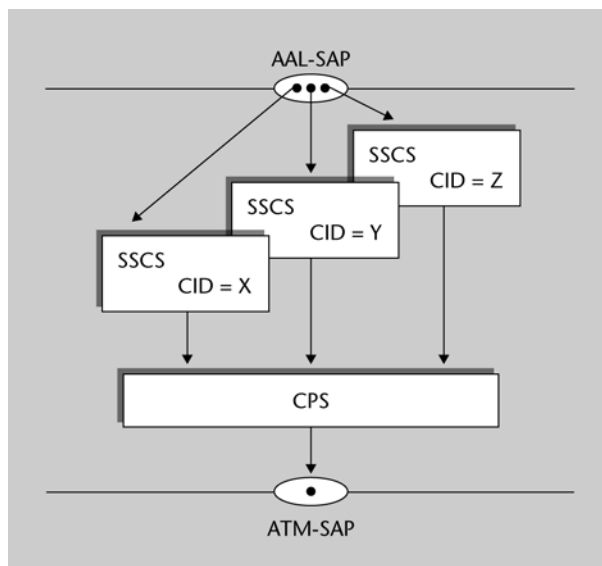
Figura 42. Model funcional d'AAL2
