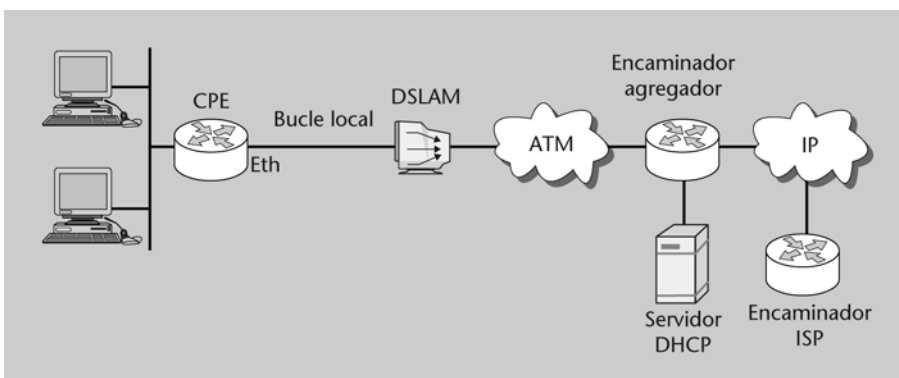
Figura 22. Components de la xarxa ADSL
