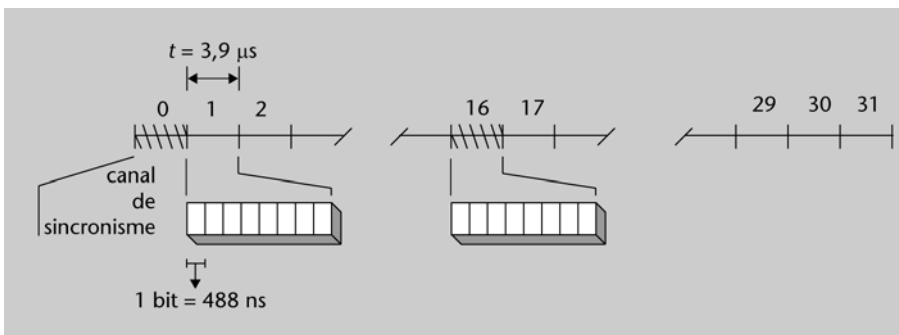
Figura 14. Representació de la trama E1
