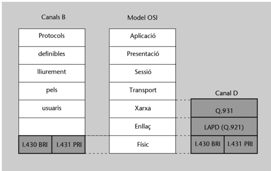
Figura 23. Equivalència entre els nivells del model OSI i l'arquitectura XDSI
