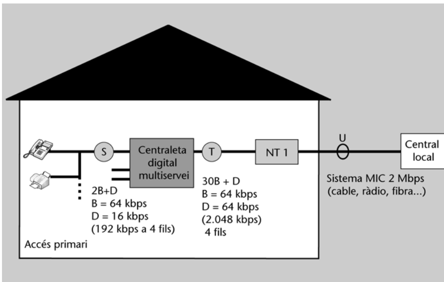
Figura 26. Accés primari (PRI) a la XDSI
