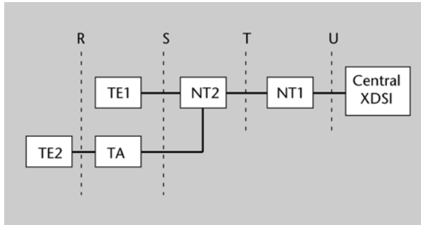
Figura 24. Configuració de referència de l'accés d'usuari a la XDSI
