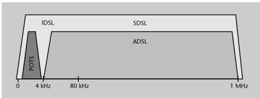
Figura 19. Assignació d'amplades de banda per a ADSL
