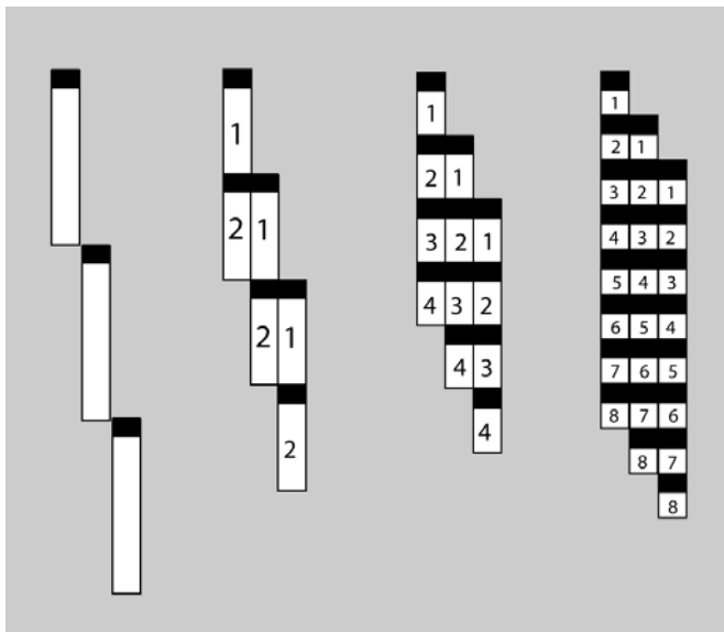
Figura 5. Temps de transmissió en funció de la longitud del paquet
