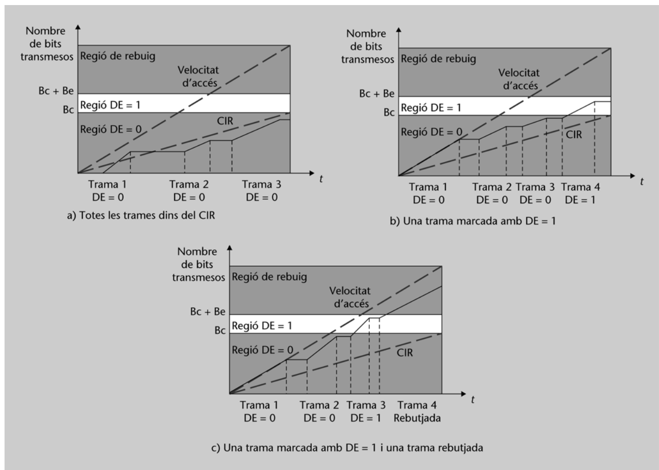
Figura 31. Exemples de gestió del trànsit
