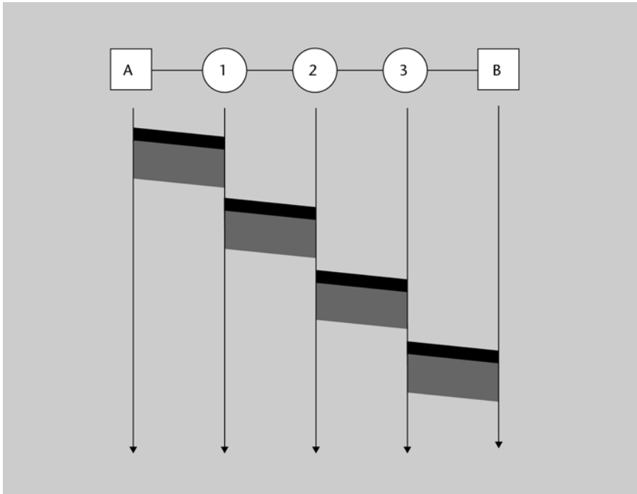
Figura 3. Diagrama temporal d'una connexió amb commutació de missatges
