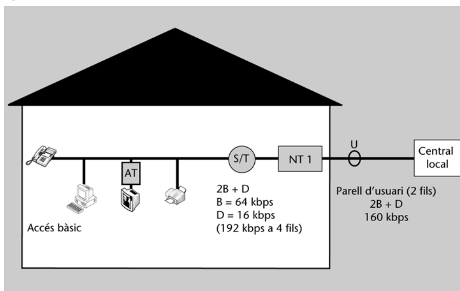
Figura 25. Accés bàsic (BRI) a la XDSI
