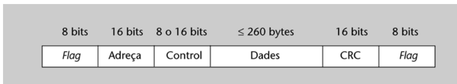
Figura 27. Estructura de la trama LAPD
