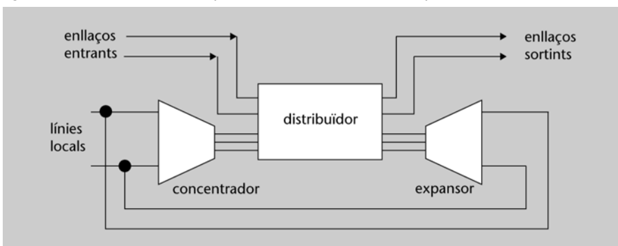
Figura 16. Commutador multietapa: concentració, distribució i expansió
