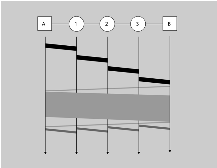
Figura 2. Diagrama temporal d'una connexió amb commutació de circuits
