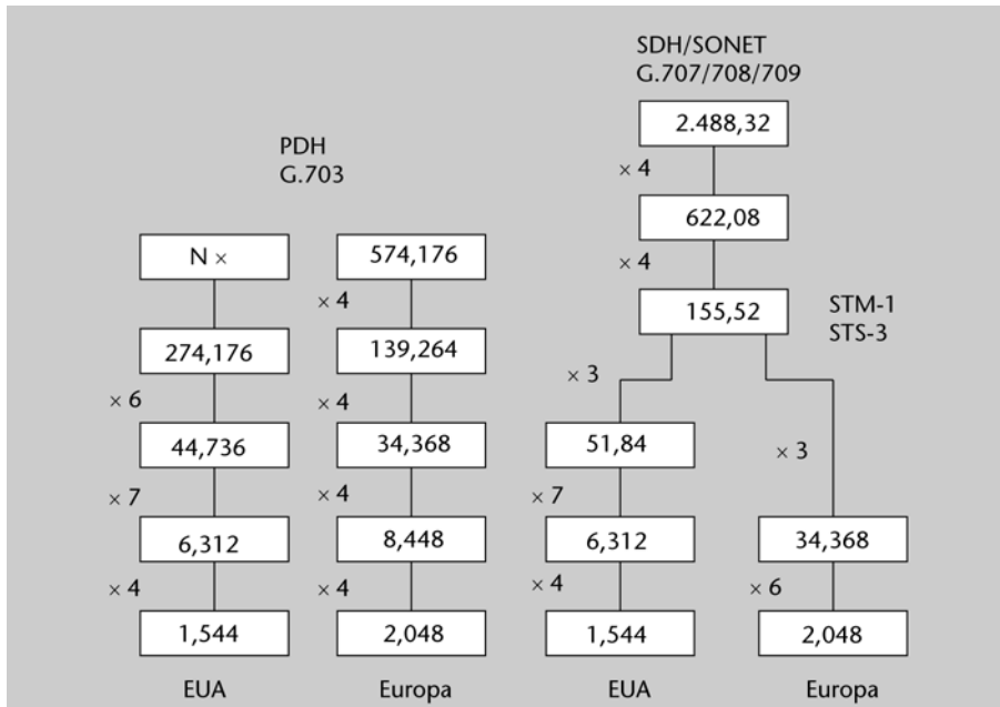
Figura 34. Esquema de les jerarquies de multiplexatge (valors expressats en Mb/s)
