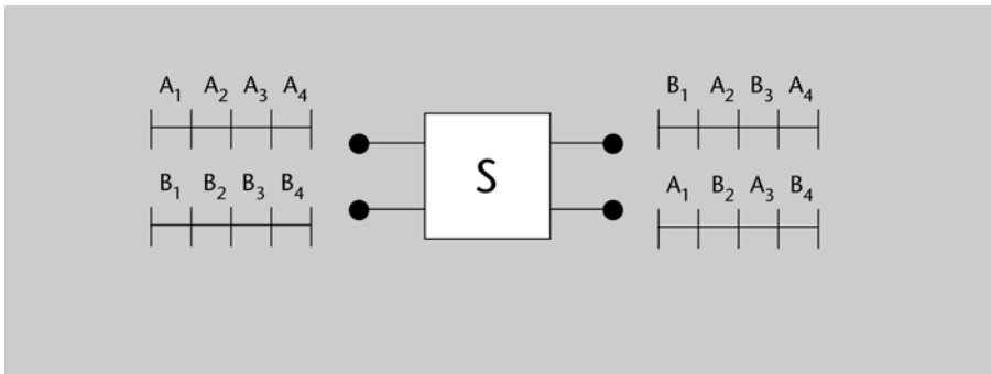
Figura 17. Commutador espacial de dues trames de quatre unitats de temps
