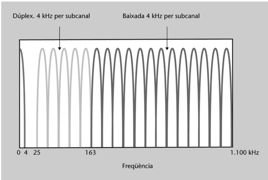
Figura 21. Assignació de subcanals per a tot el rang de freqüències
