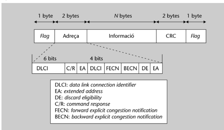
Figura 29. Format de la trama LAPF
