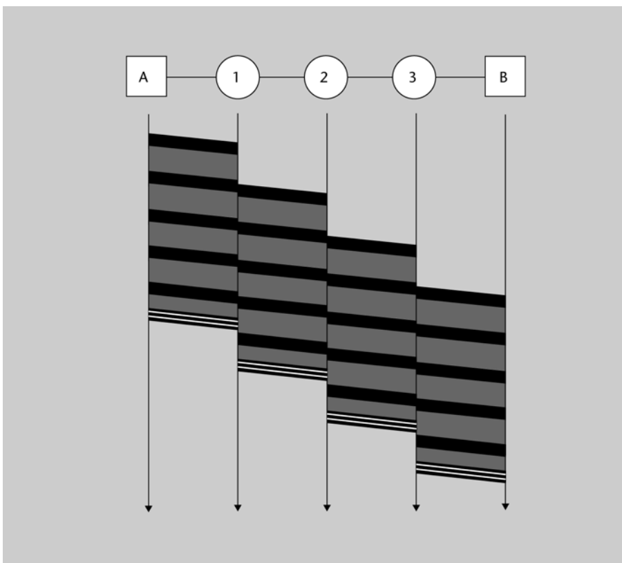
Figura 6. Diagrama temporal d'una connexió en mode datagrama
