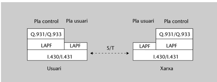
Figura 28. Protocols utilitzats a la interfície UNI
