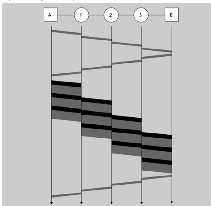
Figura 7. Diagrama temporal d'una connexió en mode circuit virtual
