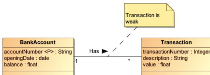
Figura 27. Exemple de tipus d'entitat dèbil ( Transaction ) i la relació identificativa amb el tipus d'entitat forta ( BankAccount )
