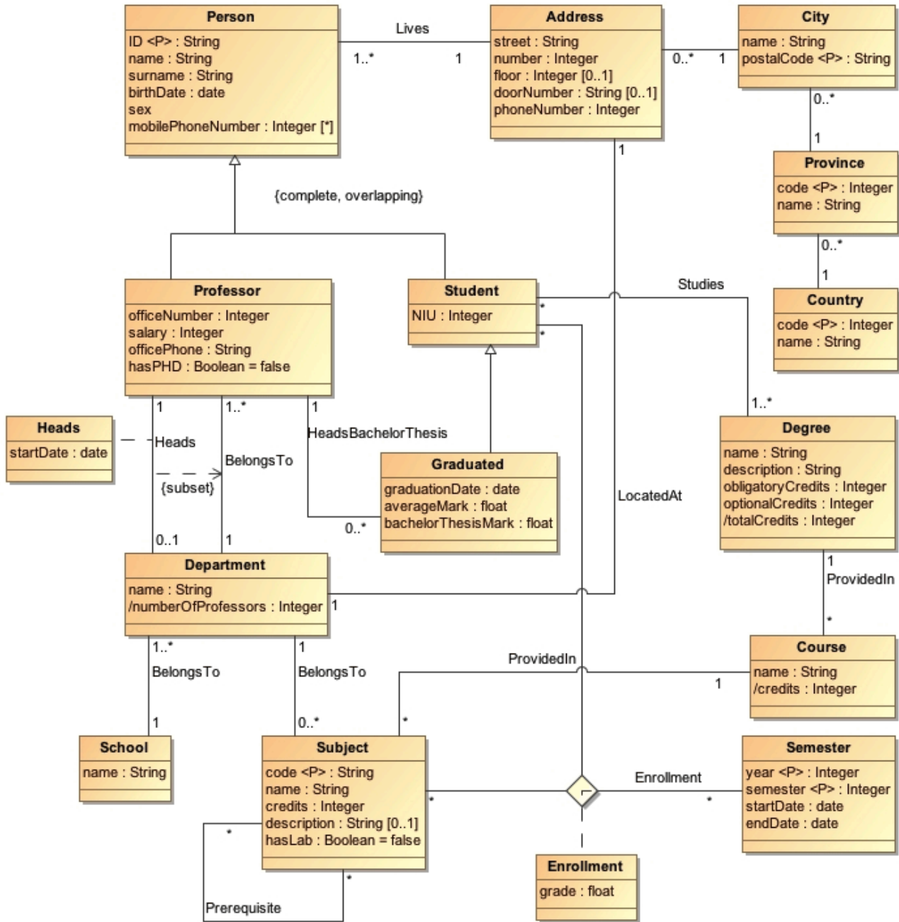
Figura 53. Diagrama del model conceptual per a la segona aproximació de la base de dades de gestió universitària
