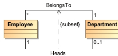
Figura 48. Exemple de restricció subset
