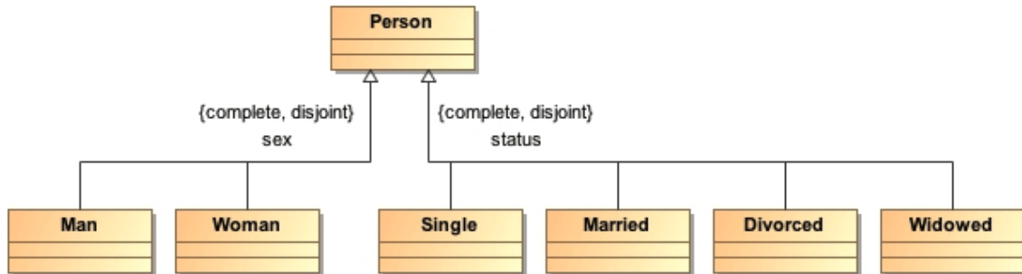
Figura 41. Exemple de generalització/especialització amb classificació múltiple
