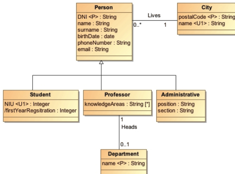
Figura 32. Exemple de generalització/especialització amb tipus de relacions
