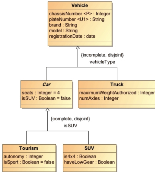
Figura 39. Exemple d'herència simple
