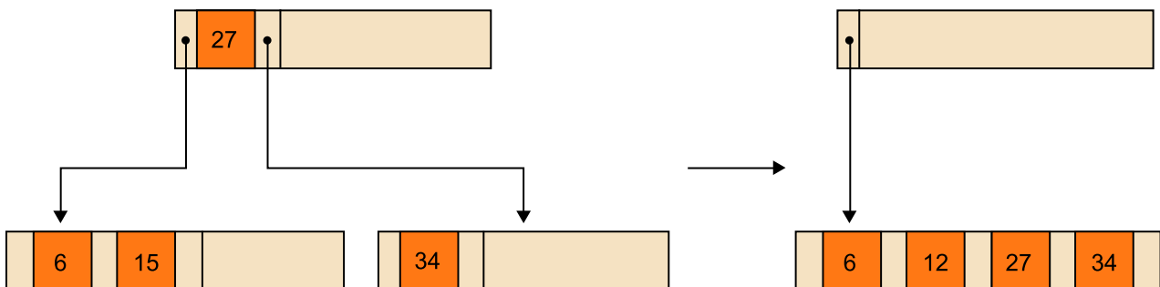
Figura 32. Fusió de nodes no-fula
