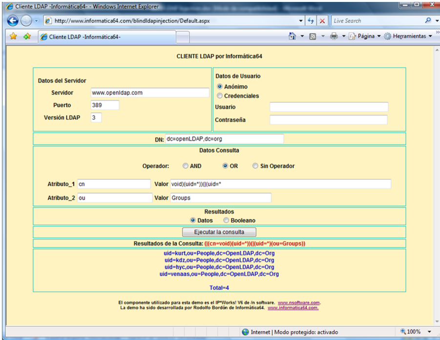
Figura 21. Lista de usuarios obtenida tras la inyección
