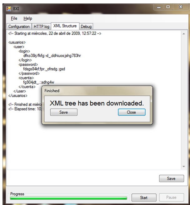
Figura 41. Árbol XML extraído mediante una aplicación automatizada
