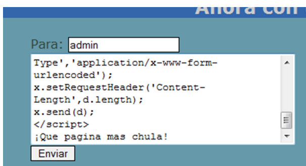
Figura 4. XSS antes de ser enviado
