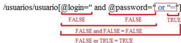
Figura 40. Evaluación de los parámetros en XPath
