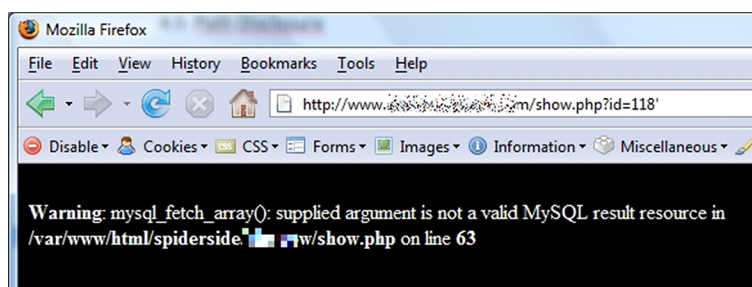
Figura 42. Fallo de Path Disclosure
