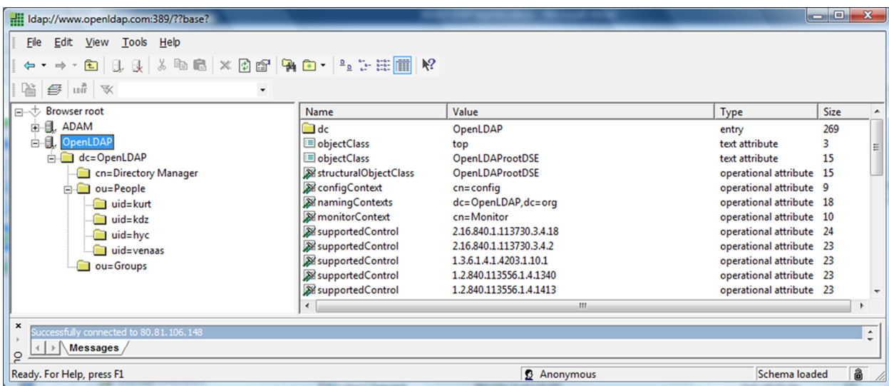
Figura 16. Estructura del árbol LDAP en OpenLDAP
