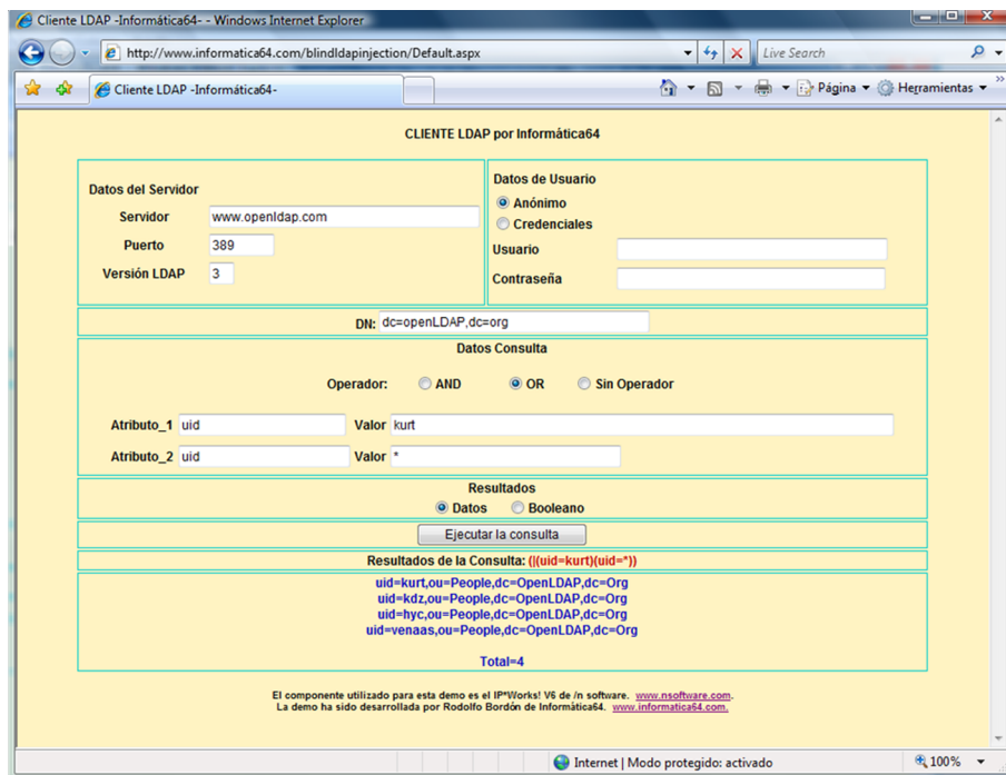
Figura 18. Todos los usuarios
