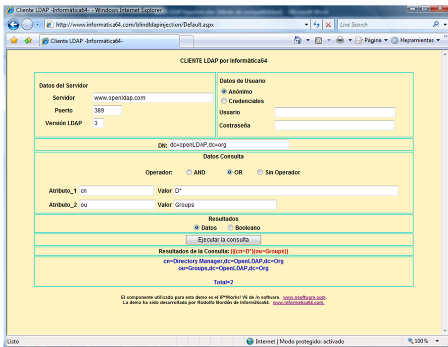
Figura 20. Consulta OR sin inyección
