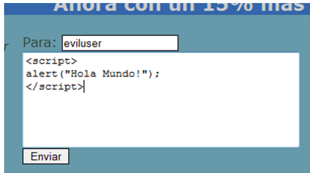
Figura 3. XSS antes de ser enviado
