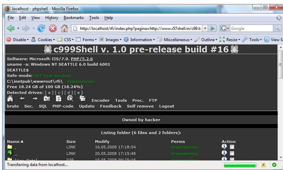
Figura 43. Shell remota ejecutándose
