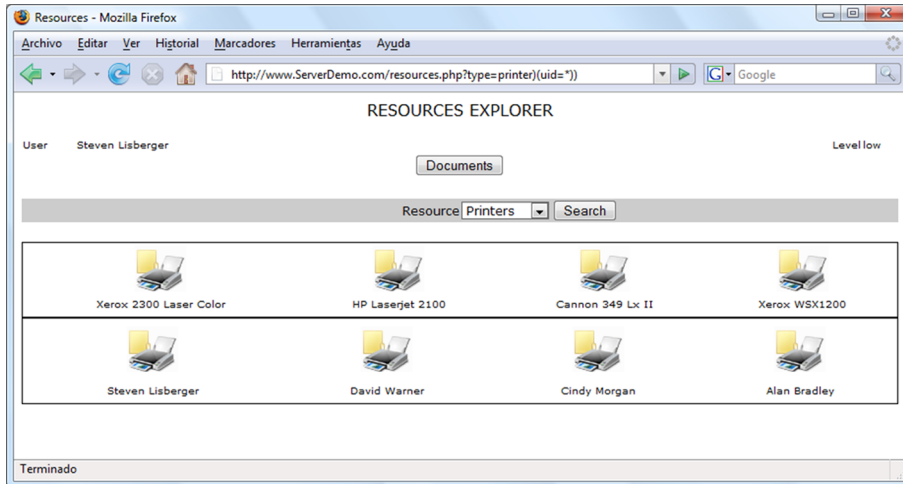
Figura 23. Acceso al listado de usuarios mediante OR LDAP Injection
