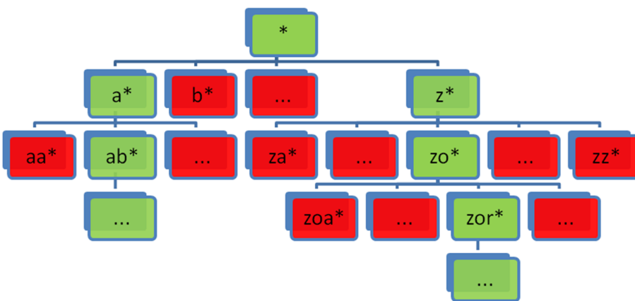
Figura 28. Árbol de despliegue. Se profundizará en todas las respuestas positivas (color verde).
