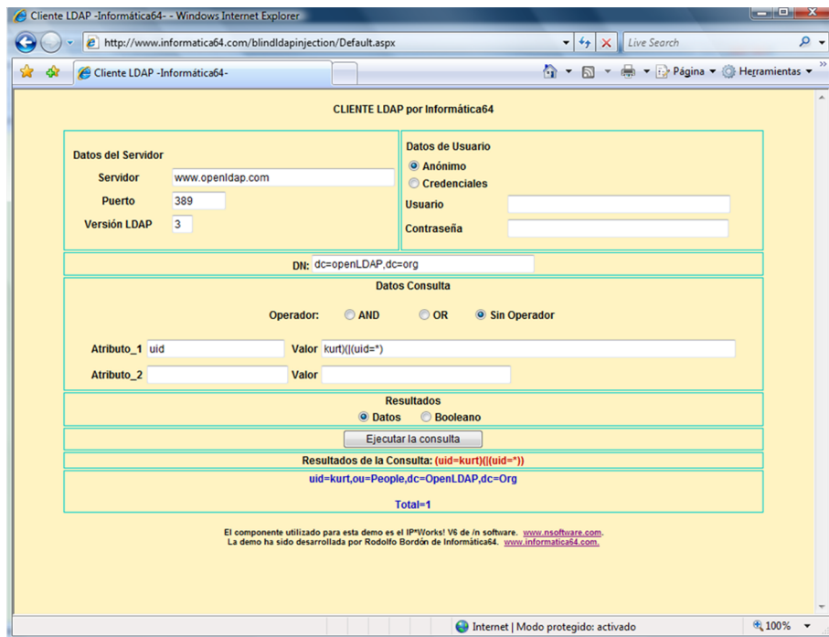
Figura 19. Inyección OpenLDAP. Se ignora el segundo filtro
