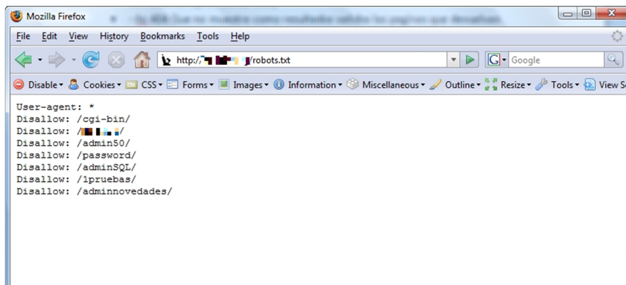
Figura 48. Ejemplo de fichero robots.txt
