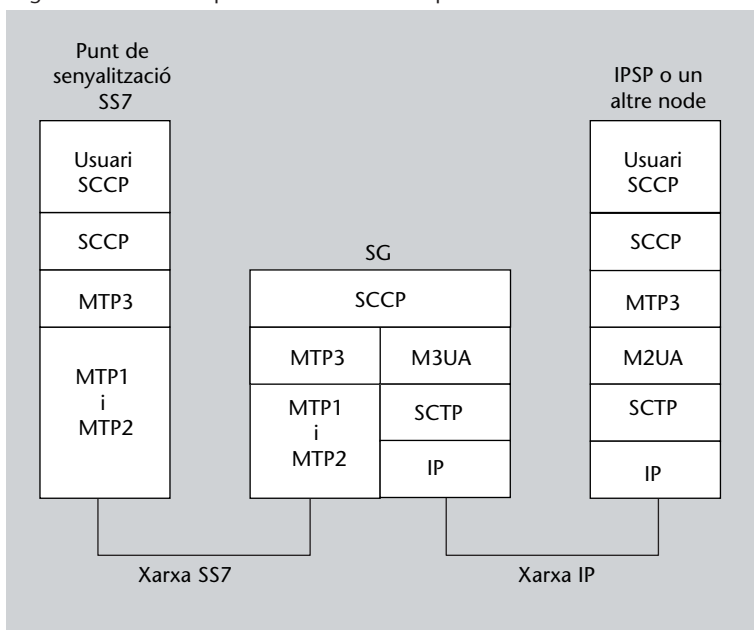
Figura 15. Tercera arquitectura de referència per a M3UA
