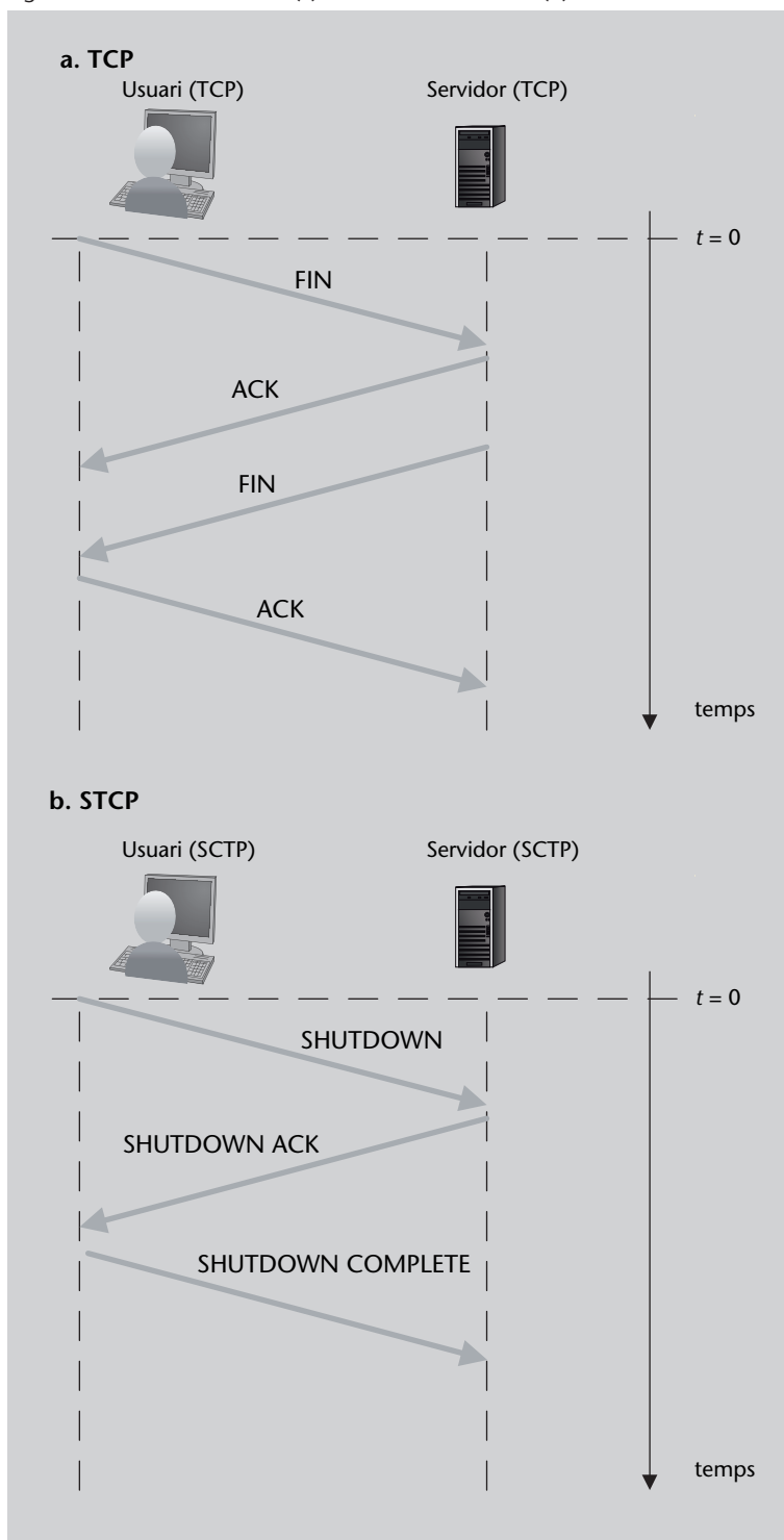
Figura 7. Alliberament d'una (a) connexió TCP i d'una (b) associació SCTP
