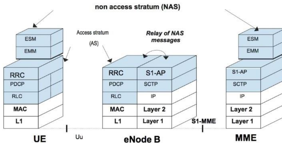
Il·lustració 119. AS, NAS i S1-AP en la pila de protocols. X. Lagrange "4G Network Essentials", Institut Mines-Télécom (Course Slides), 2018.
