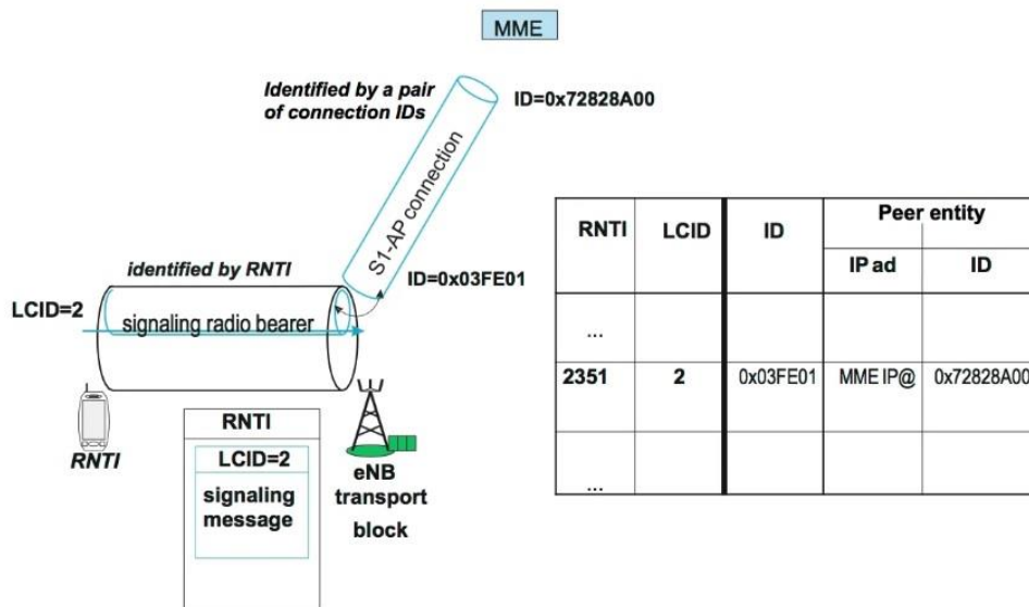
Il·lustració 116. Identificador de connexió local (ID) associat al RNTI i al LCID. X. Lagrange "4G Network Essentials", Institut Mines-Télécom (Course Slides), 2018.
