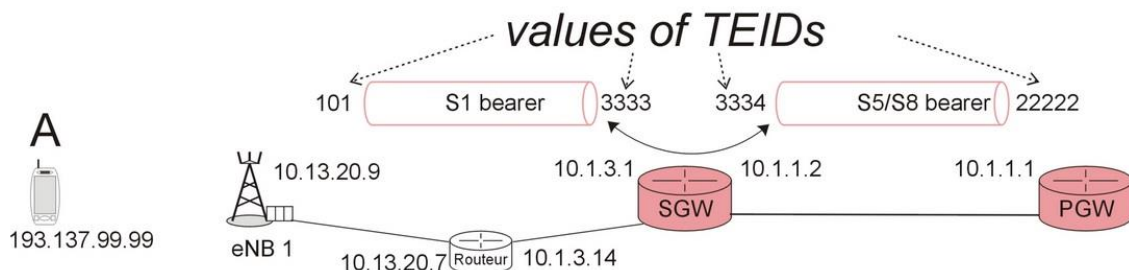
Il·lustració 112. Suposem que la xarxa està limitada als nodes que es troben presents. Només els túnels especificats estan establerts. X. Lagrange "4G Network Essentials", Institut Mines-Télécom (Course Slides), 2018.
