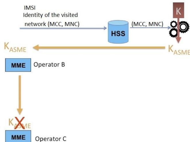
Il·lustració 52. K-ASME enviada al MME pertanyent a la xarxa que sol·licita la clau. X. Lagrange "4G Network Essentials", Institut Mines-Télécom (Course Slides), 2018.
