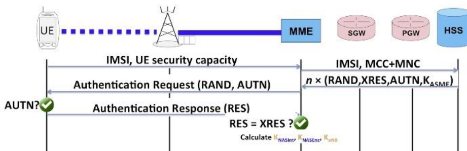
Il·lustració 60. El MME verifica que la resposta RES correspongui a XRES. X. Lagrange "4G Network Essentials", Institut Mines-Télécom (Course Slides), 2018.
