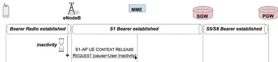
Il·lustració 137. S1-AP UE CONTEXT RELEASE REQUEST enviat pel eNodeB. X. Lagrange "4G Network Essentials", Institut Mines-Télécom (Course Slides), 2018.
