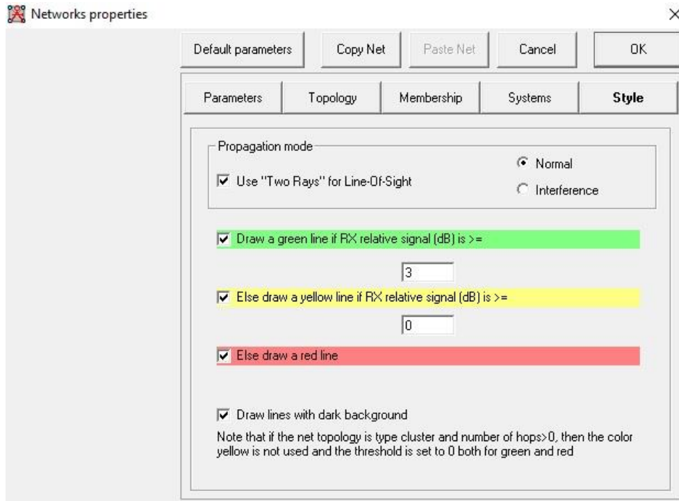
Il·lustració 198. Configuració per als llindars de recepció a Radio Mobile.
