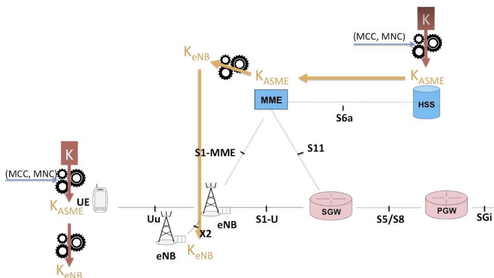
Il·lustració 53. Representació de com estan distribuïdes les claus a la xarxa. X. Lagrange "4G Network Essentials", Institut Mines-Télécom (Course Slides), 2018.
